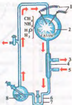
71-rasm. Miller tajribasi: 1 — elektrodlar; 2 — elektr zaryad hosil bo'lishi; 3 — suv chiqishi; 4 — sovituvcchi moslama; 5 — suv kirishi; 6 — organik moddalarni saqlovchi sovutilgan suv; 7 — sifon; 8 — qaynayotgan suv.
