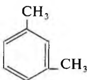
m-xilol (1,3- dimetilbenzol)
