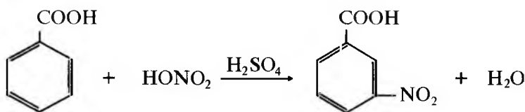
m -nitrobenzoy kislota
