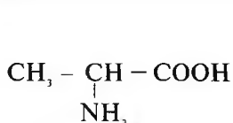
2-aminopropan kislota
