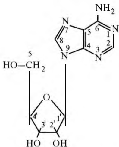
Adenozin
