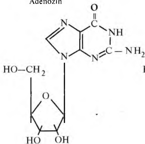
Guanozin
