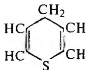
tiopiran
