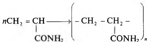
poliakrilamid
