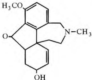
galantamin
