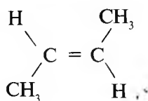
trans -2-buten
