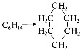
siklogeksan
