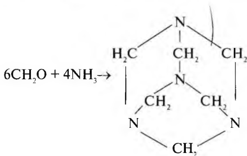
urotropin (geksametilen tetramin)
