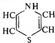
tiazin
