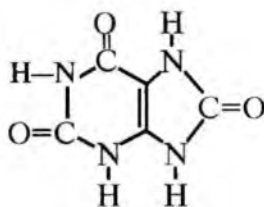
siydik kislotasi (2, 6, 7-trioksi purin)
