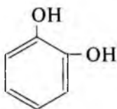
pirokatekin ( o -dioksibenzol)
