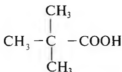
2,2- dimetilpropan kislotasi
