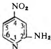
4-nitro-2-aminopiridin
