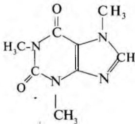
kofein
