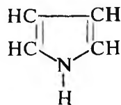
pirrol
