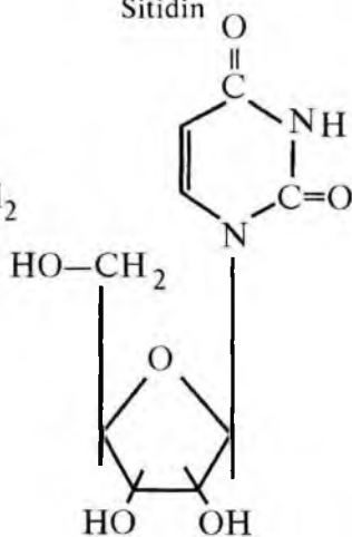
Uridin
