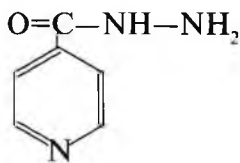
izoniazid
