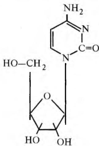
Sitidin
