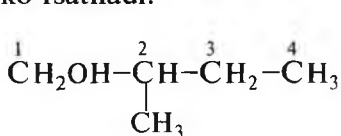
2- metilbutanol- 1
