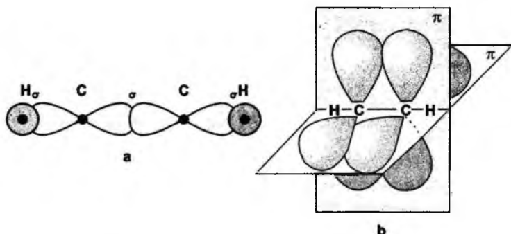
5- rasm. Asetilen molekulasida kimyoviy bog‘larning hosil bo‘lishi: a) \sigma - bog‘lar; b) \pi - bog‘lar.
