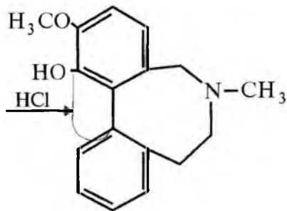
metilopogalantamin
