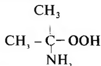
2-metil-2-aminopropan kislota
