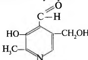
piridoksal
