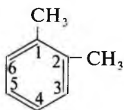
o-xilol (1,2- dimetilbenzol)
