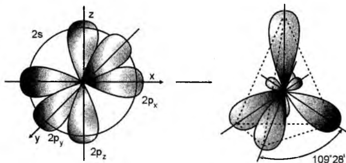
1- rasm. Uglerod atomining sp^3 - gibrilanishi.
