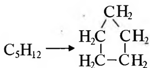
siklopentan
