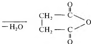
kahrabo kislota anhidridi
