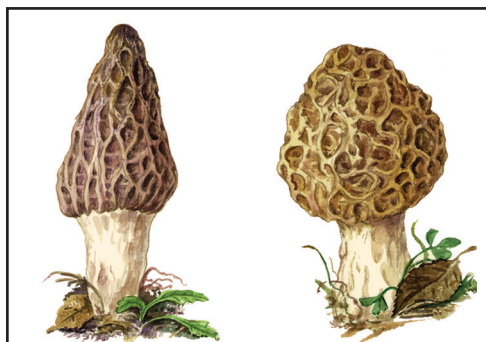
Qo'ziqorin zamburug'i.
