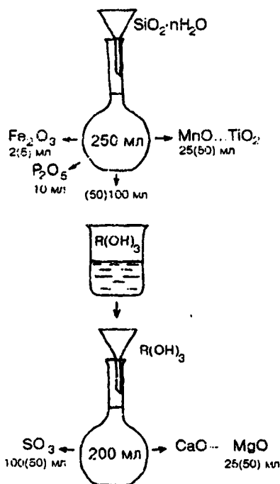
Рис. 28. Схема последовательного определения макрокомпонентов валового состава почвы из солянокислого фильтрата после отделения кремниевой кислоты.
