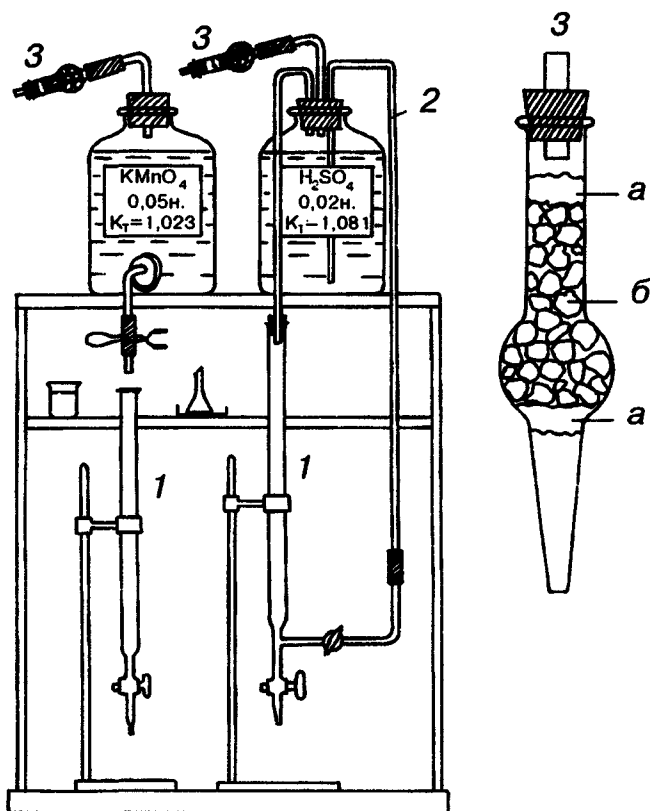
Рис. 10. Титровальная установка.
