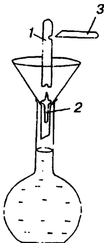
Рис. 12. Приготовление титрованного раствора из фиксанала 1 — ампула с точно известным количеством вещества; 2 — крестовидный боек; 3 — боек для пробивания отверстия в верхней части ампулы.
