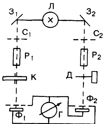
Рис. 19. Схема компенсационного фотоэлектроколориметра. Пояснения в тексте.
