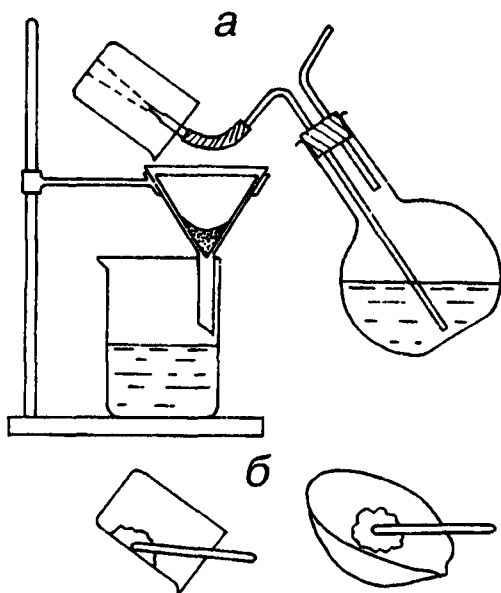
Р и с. 16. Удаление и собиpание частиц осадка.
