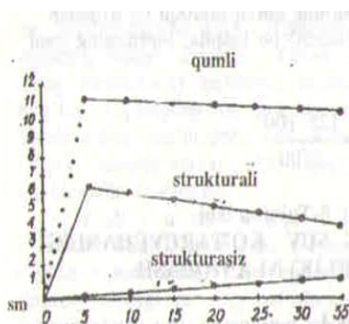
7-rasm. Qumli, strukturali va strukturasiz tuproqning suv o'tkazuvchanlik diagrammasi
