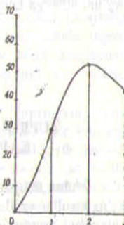
8-rasm. Tuproqning nam sig'imi diagrammasi. 1- qumli; 2- strukturali; 3- strukturasiz
