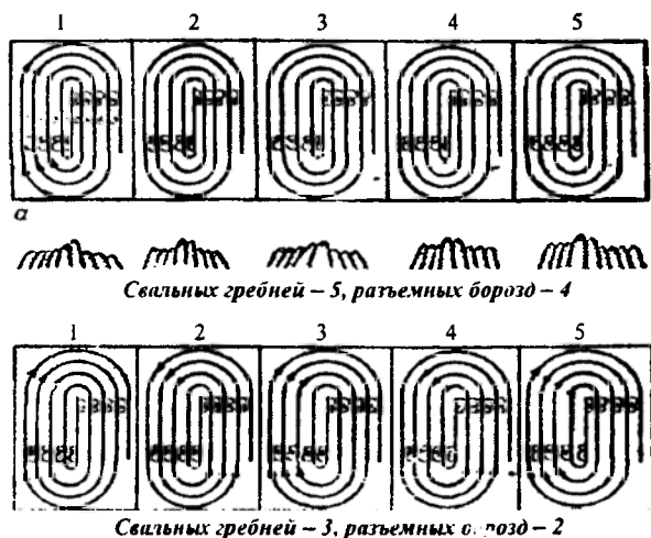
Рис.8. Схема вспашки пяти загонов.
