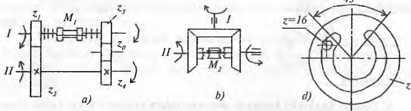
9.6-rasm. Reversiv mexanizmlar.
