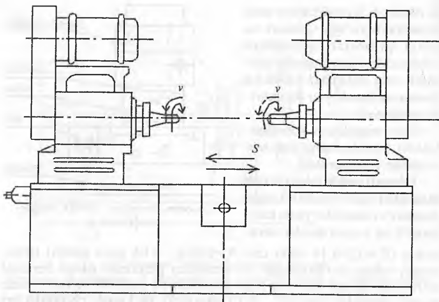
11.7-rasm. Gorizontol olmosli-teshik kengaytirish stanogi.
