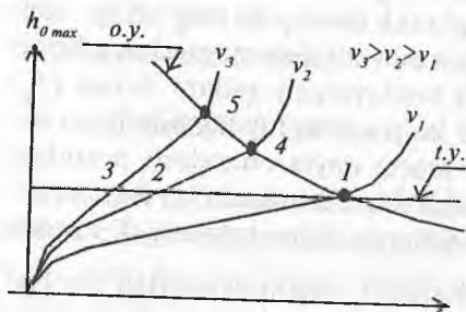
6.8-rasm. Yedirilish mezonlari.
