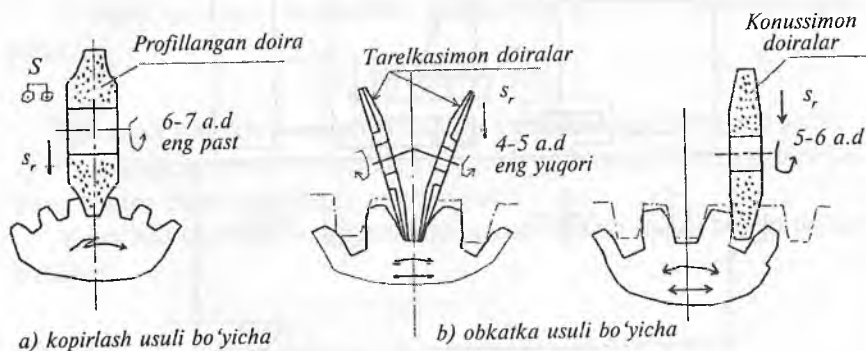
14.15-rasm. Tishlarni jilvirlash sxemalari.
