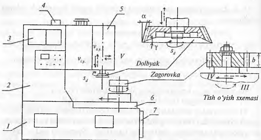
14.5-rasm. SA122 modelli tish o'yish yarim avtomati:
