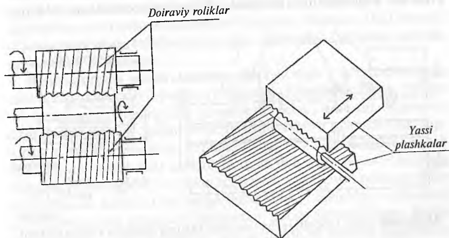
15.4-rasm. Rezbalarni nakatka qilish sxemalari.
