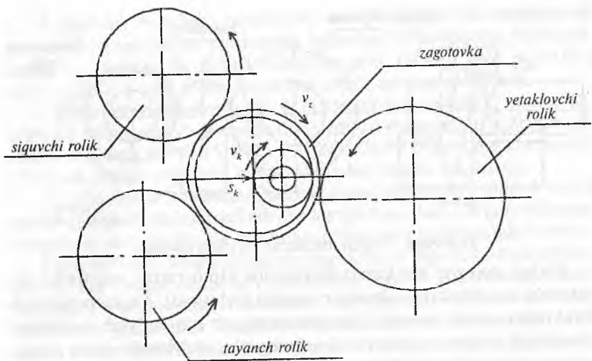
16.7-rasm. Markazsiz ichki doiraviy jilvirlash sxemasi.
