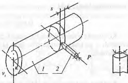
3.6-rasm. 1-qarshi jism (Cr 45 markali konstruktsion po'latdan). 2-indentor (asbobsozlik po'latidan).
