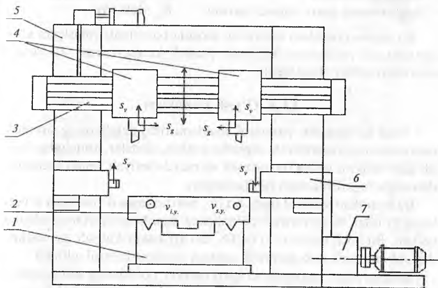
13.4-rasm. 7212 modeli ikki stoykali bo'ylama randalash stanogi. 1-stanina; 2-stol; 3-traversa; 4-vertikal supportlar; 5-portal; 6-yon supportlar; 7-stol yuritmasi
