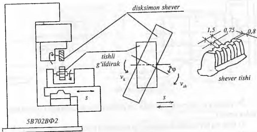
14.16-rasm. Shevinglash stanogi va shevinglash sxemasi.
