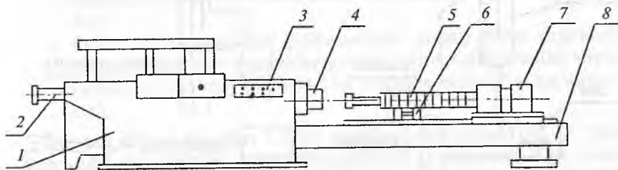
13.6-rasm. 7523 modeli gorizontol sidirish yarim avtomat stanogi: 1-asosiy stanina; 2- gidrosilindr; 3- boshqarish pulti; 4-planshayba; 5-protyajka; 6- rolik; 7- karetka; 8- qo'shimcha stanina.
