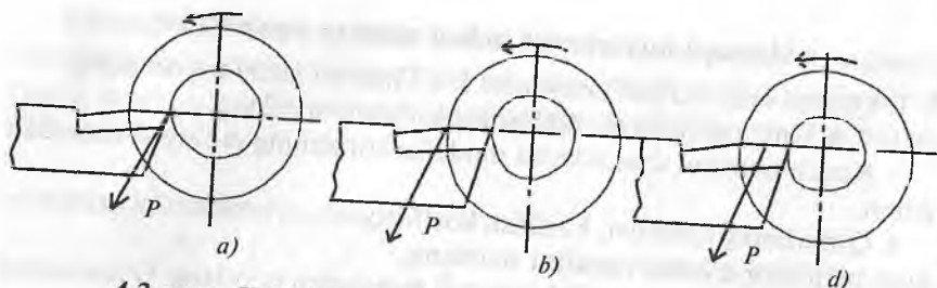
4.2-rasm. Keltirilgan kesish kuchi P_p ning asosiy kesuvchi tig'ga qo'yilish sxemasi.
