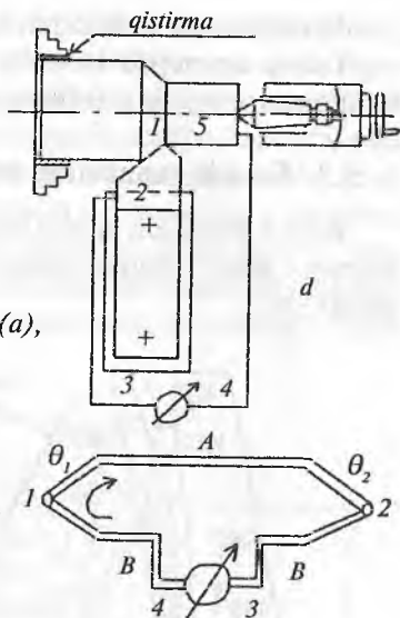
5.6-rasm. Temperaturani termojuft bilan o'lchash sxemasi.
