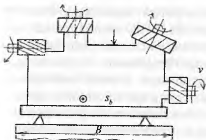
12.4-rasm. Zagotovkani frezalash sxemasi.
