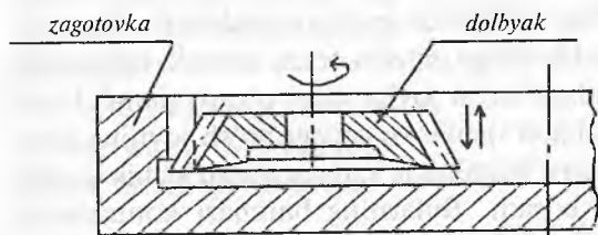
14.7-rasm. Ichki tishlarni o'yish.
