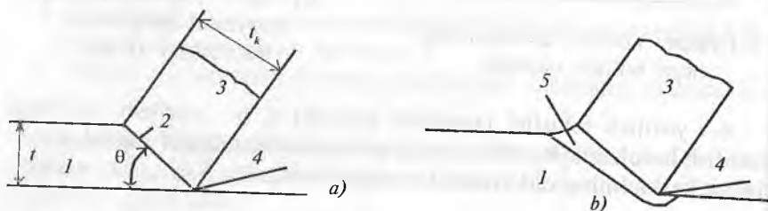
3.3-rasm. Kesishda deformatsiya zonasining sxematik tasviri: a) bir surilish tekisligiga ega bo'lgan model; b) rivojlangan zonaga ega bo'lgan model; 1-zagotovka; 2-surilish tekisligi; 3-qirindi; 4-keskich; 5-surilish zonasi; \theta -surilish (yorilish) burchagi.
