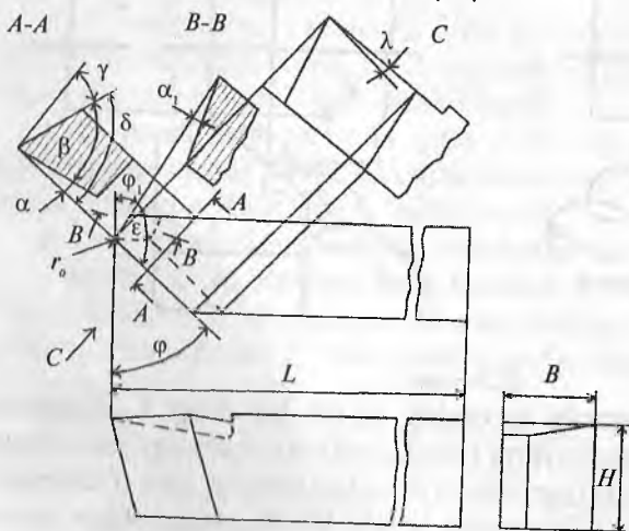
2.6-rasm. Oddiy ko'rinishdagi tokarlik keskichining chizmasi.
