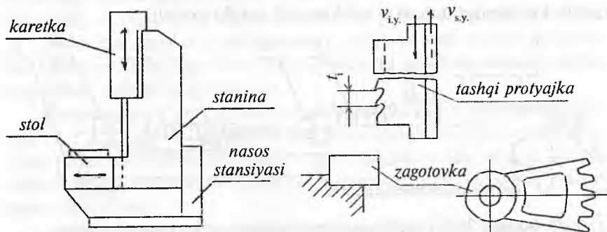
13.8-rasm. Vertikal sidirish stanogi va sidirish sxemasi.
