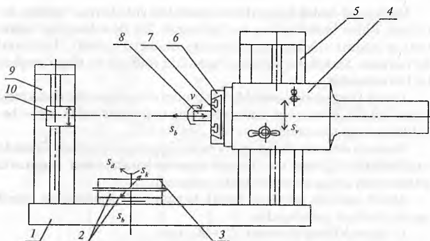
11.5-rasm. Teshik kengaytirish stanogi:
