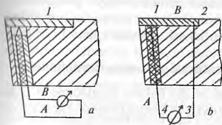
5.5-rasm. Keskichning temperaturasini sun'iy (a), yarim sun'iy (b), va tabiiy (d) termojuftlar yordamida o'lchash.
