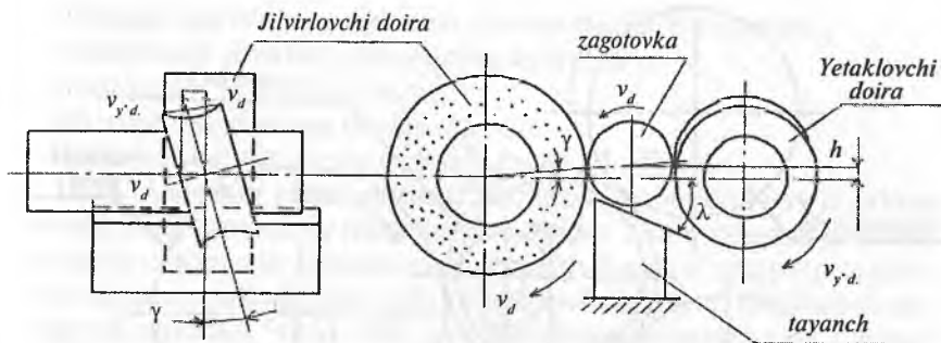
16.6-rasm. Tashqi markazsiz jilvirlash sxemasi.
