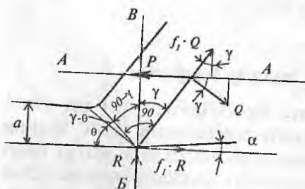
4.4-rasm. Keskich tig'iga ta'sir etuvchi kuchlar sxemasi.
