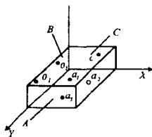
5.1-расм. Призма шаклидаги заготовкани мосламада базалаш
