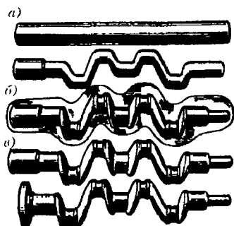
19.1-расм. Пресс ердамида штамплаш орқали тирсакли вал заготовкасининг шаклини ҳосил қилиш
