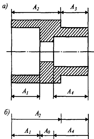
4.3-расм. Ўлчам занжирларини тузиш.
