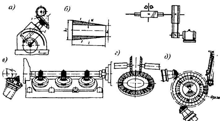
15.5-расм. Конуссимон тишли ғилдиракларда тиш фрезалаш
