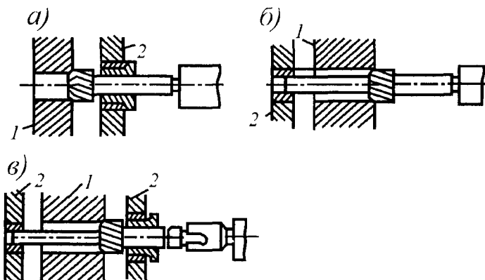
20.6-расм Корпусли деталлардаги тешикларни йўнишда асбобни йўналтирувчи таъинчилар билан ишлов бериш схемалари: а — таянч заготовка олдида; б — таянч заготовка орқасида; в — таянч заготовка олдида ва орқасида
