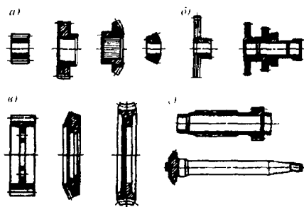
22.1-расм. Тишли филдиракларнинг асосий гуруҳлари:
