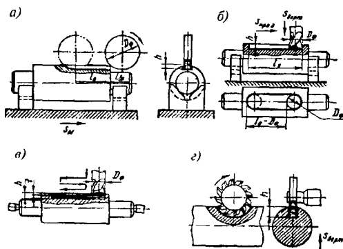
16.1-расм. Валларнинг шпонка ариқчаларини фрезалаш усуллари
