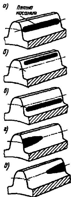
29.9-расм. Тишли филдиракларни илашишни бўёқ бўйича текширишда доғнинг кўриниши
