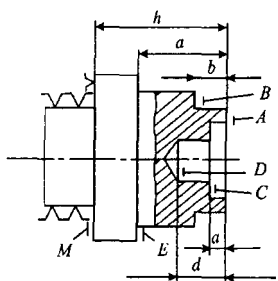
5.4-расм. Заготовкага револьверли дастгоҳда ишлов беришда A созлаш базасидан фойдаланиш
