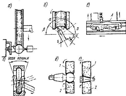
14.4-расм Шаклдор сиртларни жилвирлаш:
