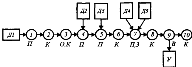
29.2-расм. Узелли автоматик йиғишнинг технологик схемаси
