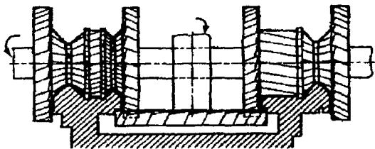
20.2-расм. Фрезалар тўплами ердамида дастгоҳ станиналарининг йўналтирувчиларини фрезалаш схемаси
