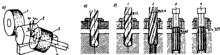
11.1-расм. Яхлит материалда тешикка ишлов бериш:
