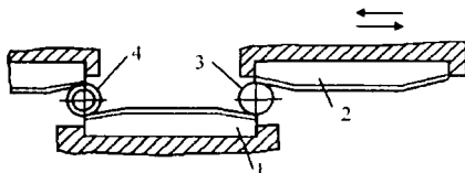
12.5-расм. Ясси думаловчи плашкалар ёрдамида резба ўйиш
