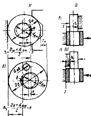
29 3-расм. Валик ва втулкаи автоматик йиғишда бикир базалаш
