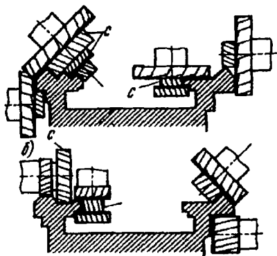
20.3-расм. Саккиз шпинделли бўйлама-фрезалаш дастгоҳида дастгоҳ санина-ларининг йўналтирувчисига ишлов бериш схемаси
