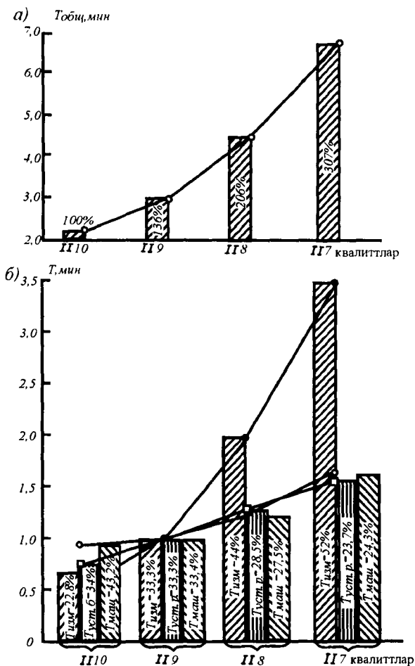
7.2-расм. Ишлов бериш иш ҳажмининг талаб қилинган аниқликка боғлиқлиги: а-умумий сарфланган вақт- T_{\text{ум}} ; б-сарфланган вақтнинг алоҳида элементлари, T_{\text{маш}} -машинали (асосий) вақт, T_{\text{уст.р.}} -кескични ўрнатиш учун сарфланган вақт, T_{\text{уст.б.}} -ўлчаш учун сарфланган вақт
