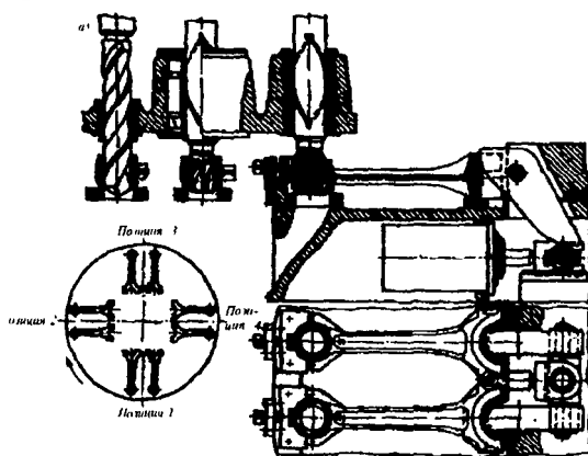
21.4-расм. Тешиқларга ишлов бериш схемаси
