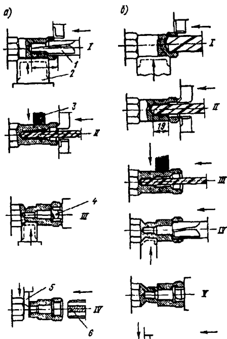
17.9-рasm. Двигател свечасининг корпусига ишлов бериш учун тырт ва олти шпинделли автоматни созлаш
