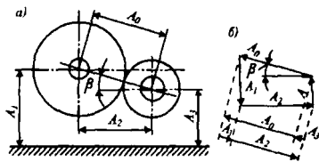
4.2-расм. Ясси ўлчам занжирини чизиқли ўлчам занжирига келтириш.
