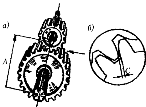
29.8-расм. Эволвентли тишли жуфтликни йиғиш-ни текшириш
