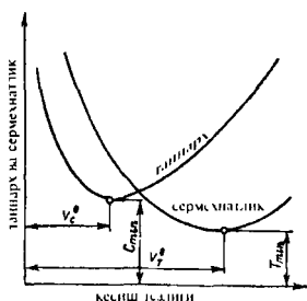
7.3-расм. Кесиш тезлигига ишлов бериш иш ҳажмининг ва таннархнинг боғлиқлиги
