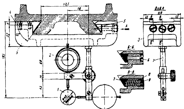
28.2-расм. Консолли фрезалаш дастгоҳи ҳартуми ҳолатининг шпиндель ўқиға нисбатан параллелигини назорат қилиш мосламаси
