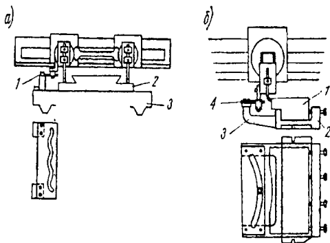
14.3-расм. Нусхакаш ердамида шаклдор сиртларни рандалаш: а — дастгоҳ столига ўрнатилган; б — кронштейнга маҳкамланган
