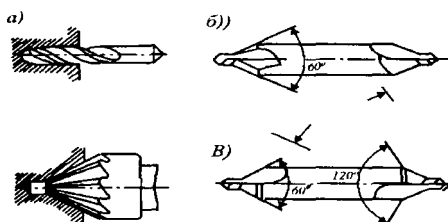
9.5-расм. Марказлаш ва марказловчи пармалар
