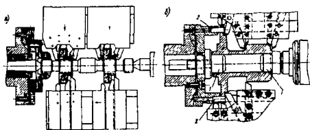
17.5-расм. Кўп кескичли ярим автоматни ишлов бериш учун созлаш
