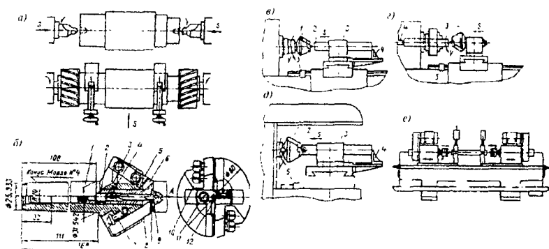
9.6-расм. Марказлаштириш схемалари:
