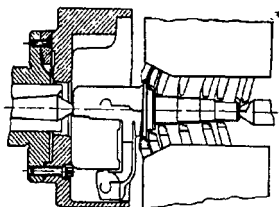
17.6-расм. Буровчи кулакни ишлов бериш учун созлаш
