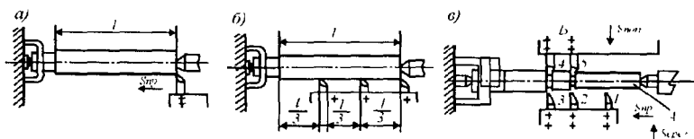
10.1-расм. Вал йўниш схемалари
