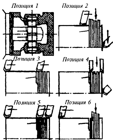
21.7-расм. Поршенни йўниш учун олти шпинделли токарлик ярим автоматни созлаш схемаси
