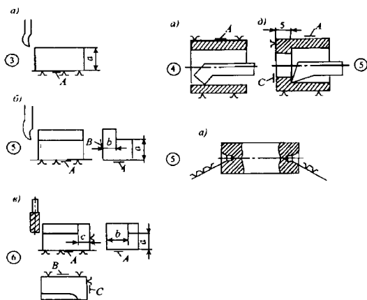
5.3-расм. Заготовкарга ишлов беришда битта (а, г), иккита (б, д, е) ва учта (в) базалардан фойдаланиш
