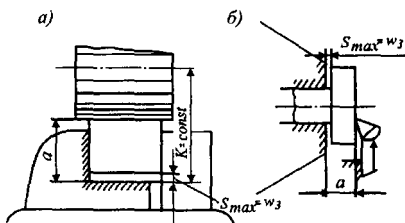
2.14-рasm. Фрезалашда (а) ва токарлик ишлов беришда (б) маҳкамлаш хатолиги \omega_{max} = S_{max}
