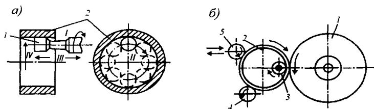
11.4-расм. Тешикларни жилвирлаш схемаси: а — планетарли; б — марказсиз
