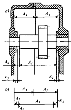
4.5-расм. Тишли узатманинг ажрайдиган корпусининг чизиқли ўлчамлари
