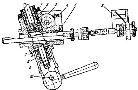
10.3-расм. Поғонали валларни йўниш учун ярим автомат мосламанинг конструкцияси
