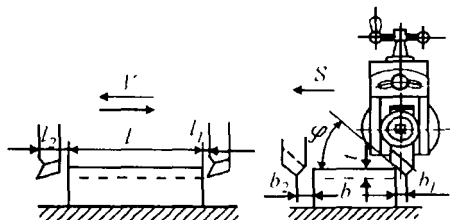
13.1-расм. Ясси сиртни рандалаш схемаси
