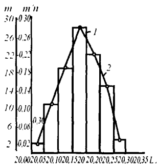
2.6-расм. Заготовкларнинг аппикланган ўлчамларининг тақсимланиши
