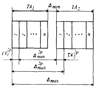
27.1-расм Гуруҳли допускли аниқлаш схемаси
