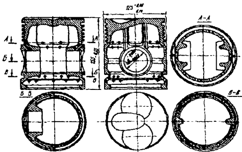
21.5-рasm. Двигатель поршени a — дизел еқилғили тракторники; б — снгил автомобилники
