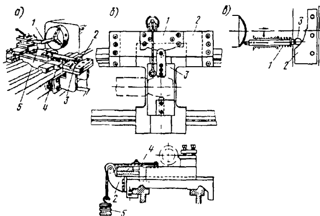
14.1-расм Нусхакаш бўйича шаклдор сиртларни йўниш а — тортқиға маҳкамланган ролик, б — юкли ролик, в — пружинали ролик.
