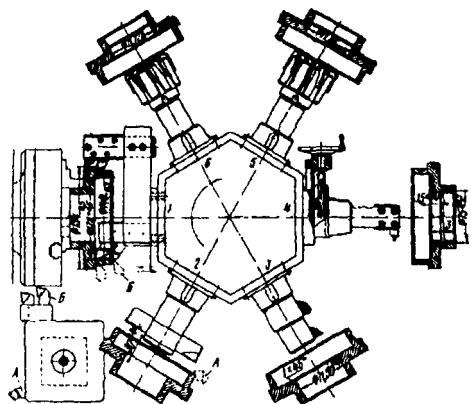
22 2-расм. Револьверли дастгоҳда тишли филдиракка ишлов бериш учун технологик созлаш
