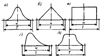
2.15-расм. Ўлчамларнинг гурли тақсимланиш қонунлари учун хомакиларга нуқсонсиз ишлов бериш шарти
