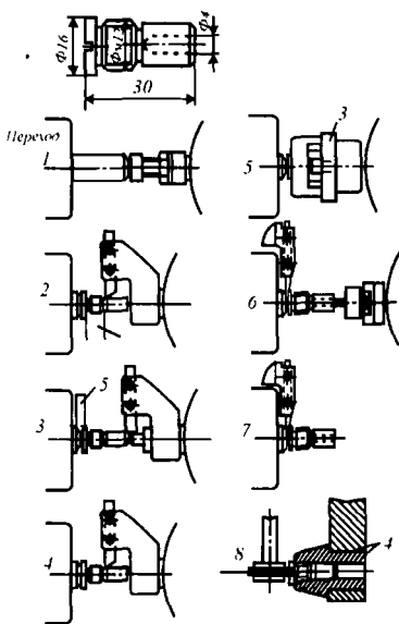
17.8-расм. М12 диаметри винтга ишлов бериш учун токарлик-револьверли автоматни созлаш схемаси
