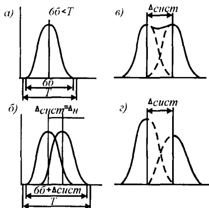
2.11-рasm. Заготовкарларнинг бир нечта партиясига дастгоҳни қайта соzлаш билан ишлов беришда Δмунт таъсири натижасида тасодикий хатоликларнинг йиғинди эгри чизиги шаклининг ўзгариши.
