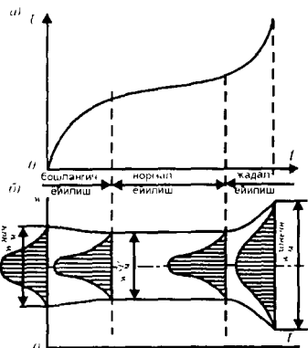
2.12-рasm Кесувчи асбобнинг ёйилиши (а) ва ишлов берилган заготовкалар ўлчамларининг оний ёйилиш майдонининг ўзгариши (б)
