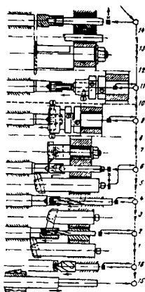
17.4-расм. I тур дастгоҳи револьверли каллагини созлаш
