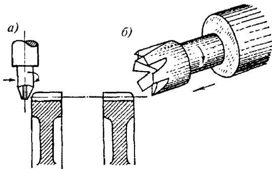
15.6-рasm. Цилиндрик тишли ғилдиракларнинг тишларини думалоқлаш
