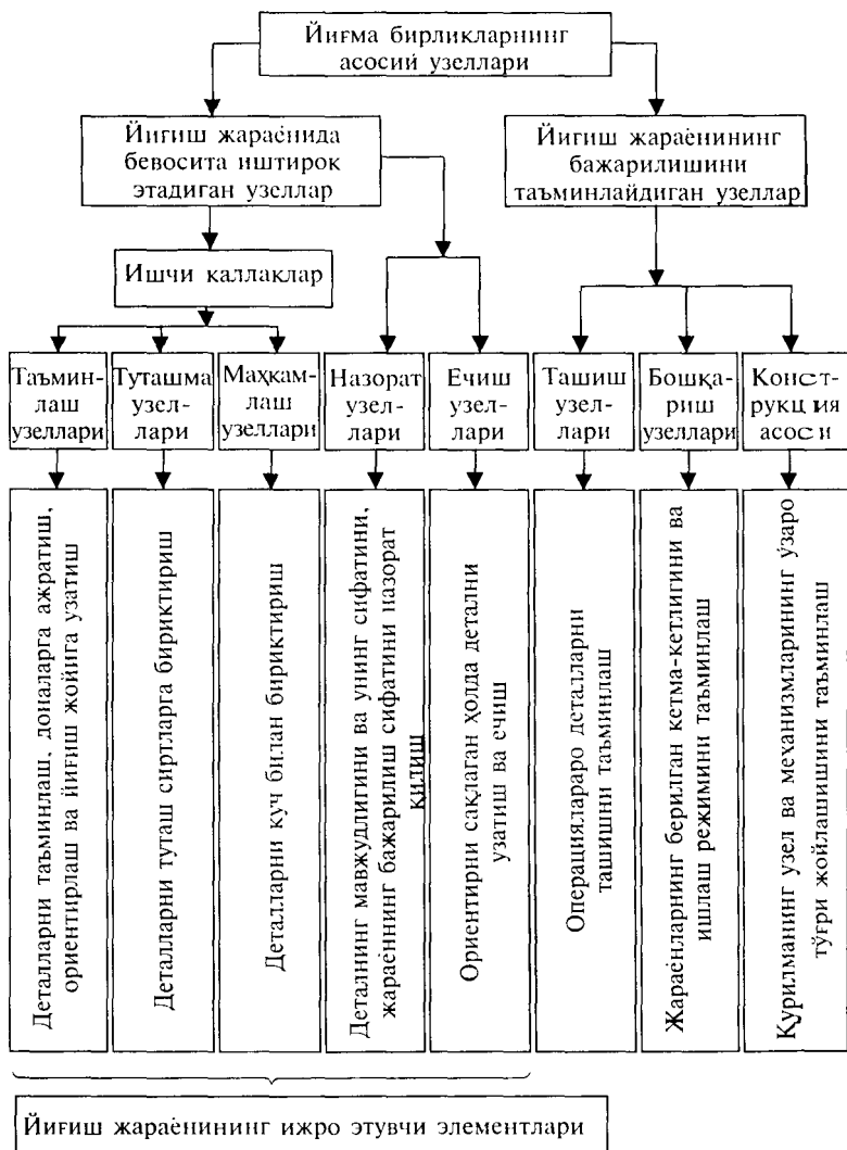
29.1-расм. Автоматлаштирилган йиғиш учун жиҳозларни яратишда ҳал қилинадиган масалалар схемасининг структураси
