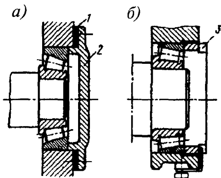
29.7-расм. Конуссимон роликли подшипникда тирқишни созлаш усуллари
