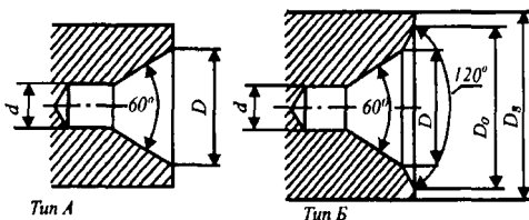
9.4-расм Марказий тешиklar
