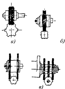
16.3-расм. Валларнинг шлицаларининг пардозлашнинг усуллари
