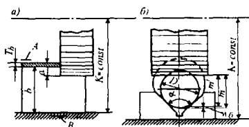
2.13-рasm Базалаш хатолиги \omega_D = \omega_6 нинг келиб чиқиши
