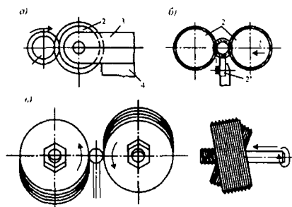
12.6-расм. Роликлар ёрдамида резба ўйиш:
