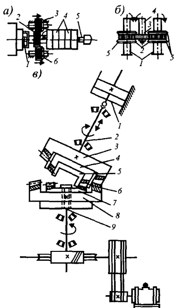
15.7-расм. Тишли гилдиракларнинг тишларини думалатиб ўйиш
