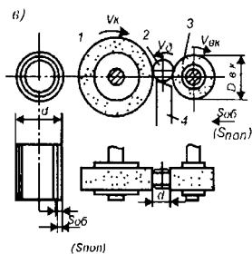
10.5-расм. Марказсиз жилвирлаш схемалари: а—умумий схемаси; б—бўйлама суриш орқали жилвирлаш; в—кўндаланг суриш орқали жилвирлаш, 1—жилвиртош доираси, 2—ишлов бериладиган детал, 3—стакловчи жилвиртош доираси; 4—таянч (пичоқ)
