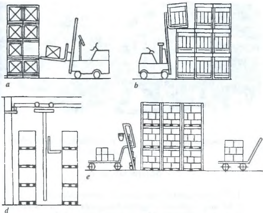
32 - rasm. Omborlarda ba'zi yuklarni saqlash sxemasi: a,b va d-mexanizatsiyalashgan variant, e-kichik mexanizatsiyalashgan variant
