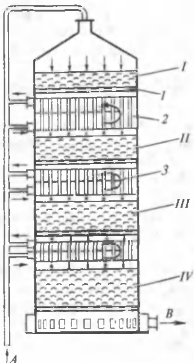
36- rasm. Qavatlari orasida issiqlik almashtirgichi bo'lgan tokchali kontakt apparati.
