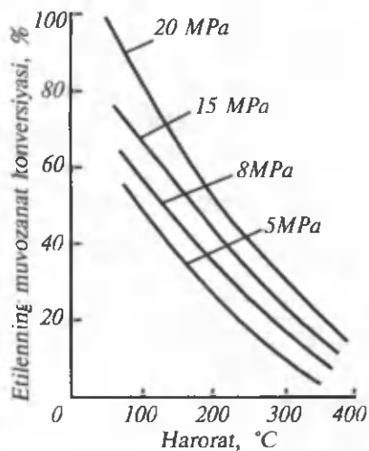
105- rasml. Etilenni spirtga etanolga aylanishdagi muvozanat konversiyasining harorat va bosimga bog'liqligi.
