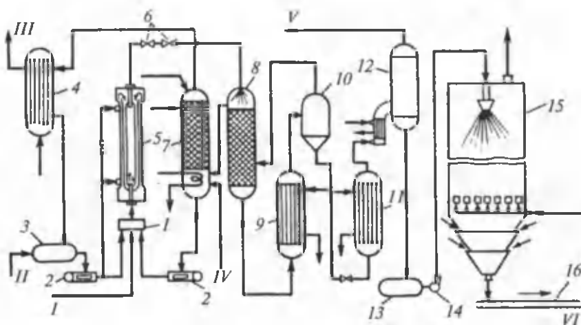
72- rasmi. Karbamid ishlab chiqarishning sxemasi.
