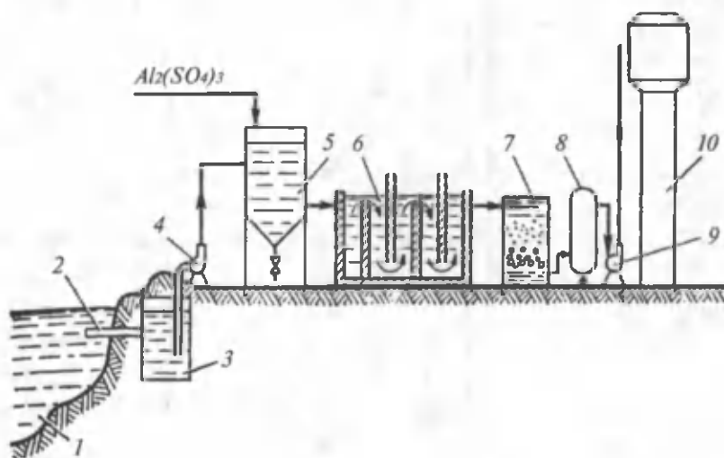
12- rasm. Ichimlik suvini tayyorlash sxemasi.
