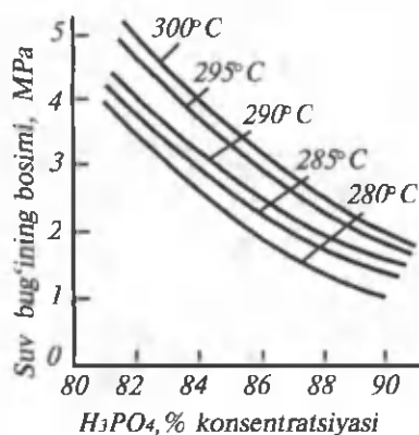
106- rasml. Turli haroratlarda suv bug'i bosimining fosfat kislot konsentratsiyasiga bog'liqligi.
