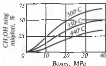
102- rasml. Reaksiya aralashmada metanolning muvozanat ulushining (miqdorining) bosim va haroratga bog'liqligi.
