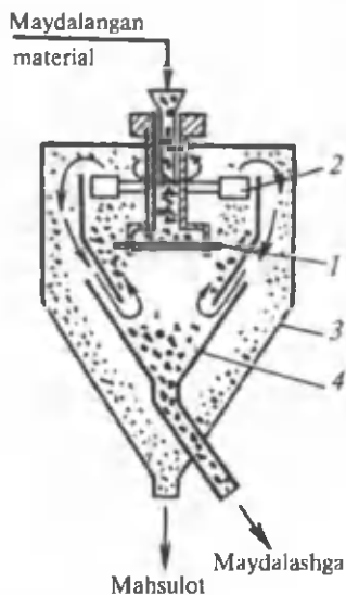
4- rasm. Havo separatori sxemasi.
