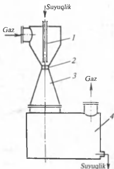
45- rasmi. Venturi apparati.
