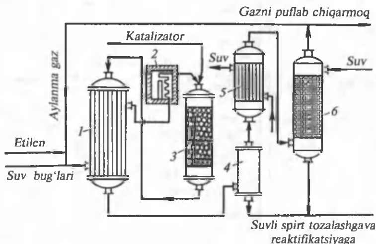
107- rasm. Etanol ishlab chiqarish uchun etilenni bug'li muhitda katalitik gidratlash qurulmasining sxemasi.
