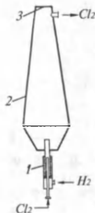
43- rasm. Vodorod xloridni sintezlash pechi.
