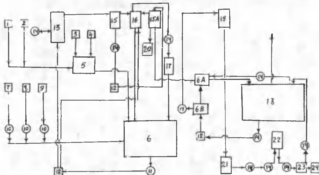
119- rasm. Nitron ishlab chiqarish sxemasi.
