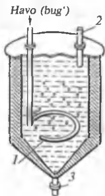
32- rasm. Pnevmatik aralashtiruvchi reaktor. 1 — barbatyor; 2 — havo chiqadigan va suyuqlik solinadigan teshigi; 3 — mahsulotning chiqishi.
