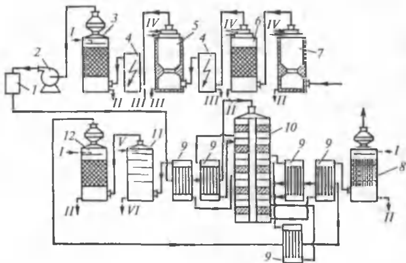
61- rasm. Kolchedanni kuydirib olingan gazdan ( \text{SO}_2 ) sulfat kislota ishlab chiqarishning taxminiy IK/IA sxemasi.
