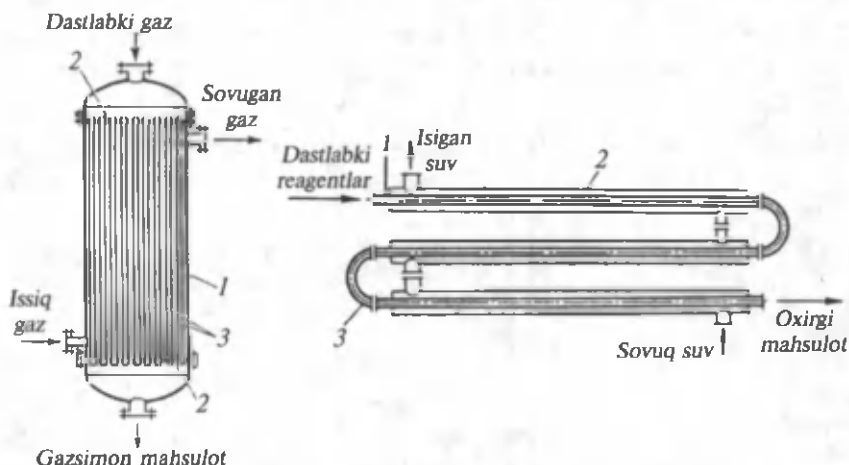
44- rasm. Quvurg'iloqli issiqlik almashtirgich apparati.
