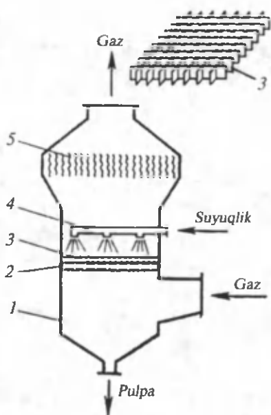
46- rasm. Ko'pik hosil qiluvchi apparat.
