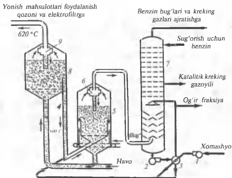
99- rasm. Katalizatori qo'zg'alib turuvchi reaktorda katalitik krekning sxemasi.
