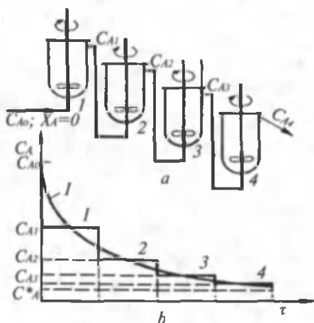
35 a, b- rasm. Ketma-ket ulangan to'liq aralashtirish reaktorlari.
