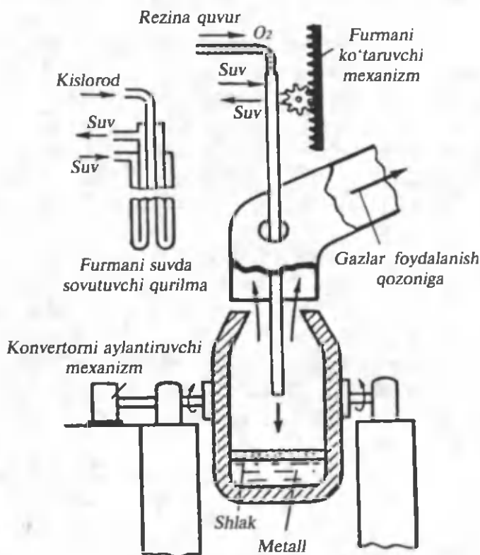
87- rasm. Po'lat eritish uchun kislorod konvertori.
