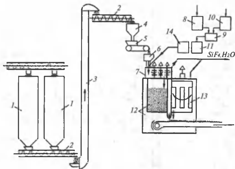
74- rasm. Uzluksiz usulda superfosfat ishlab chiqarish sxemasi.
