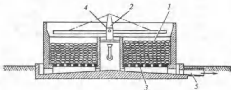
16- rasm. Aylanuvchi sachratgichli biologik filtrning sxemasi.
