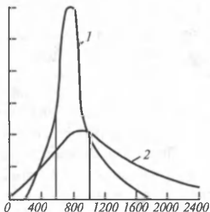
110- rasm. Polimerlarda molekularlarning molekular massalari bo'yicha taqsimlanishi. 1 — nitrosellyuloza; 2 — polistirol.
