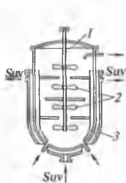
31- rasm. Parrakli aralashtirgichi bo'lgan reaktor. 1 — o'q(val); 2 — aralashtirgich; 3 — suv ko'ylagi (g'ilofi).
