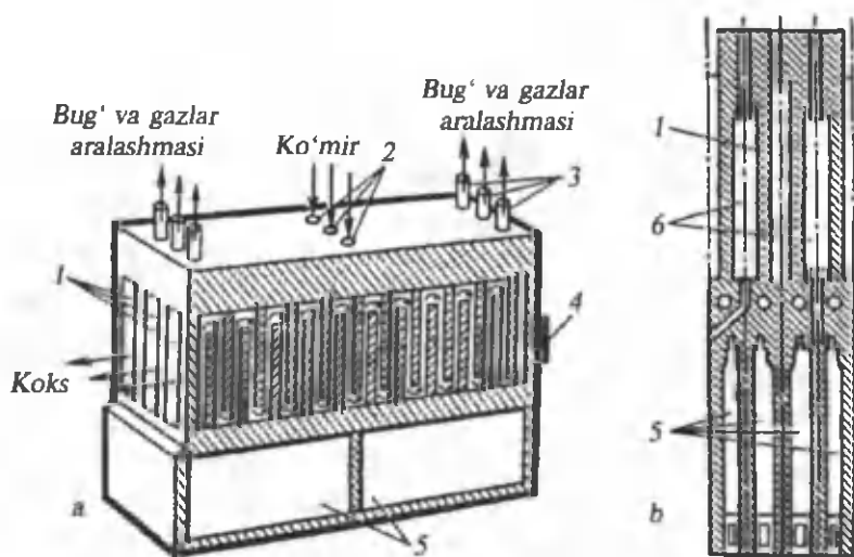
90- rasn. Koks batareyasi.
