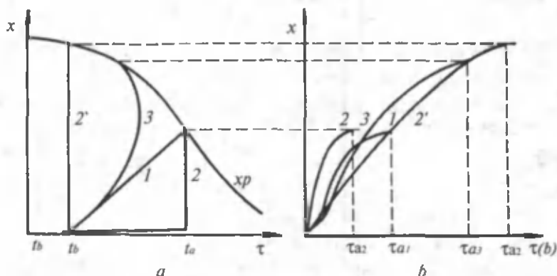
34- rasm. Adiabatik va politermik siqib chiqarish reaktorlarining harorat tartiblarini iztermik to'liq aralashtirish reaktorlari harorat tartiblari bilan taqqoslash(a). Turli reaktor tiplarida dastlabki moddaning mahsulotga aylanish darajasining vaqtga bog'liqligi(b).
