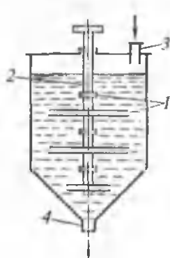
33- rasm. Varrakli aralashtirgichi bo'lgan reaktor. 1 — varragi; 2 — o'q(val); 3 — dastlabki modda solinadigan joyi; 4 — mahsulot chiqariladigan joyi.
