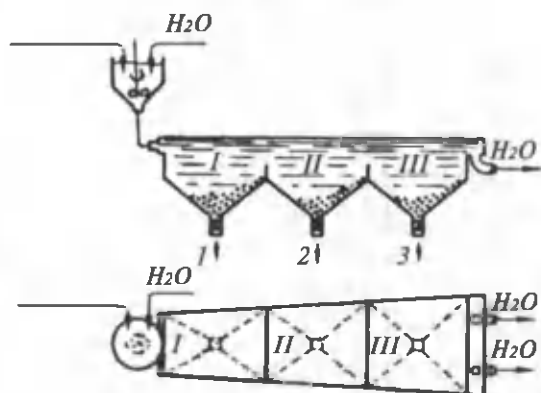
5- rasm. Ho'l usulda gravitatsion boyituvchi cho'ktirish mashinasining sxemasi.
