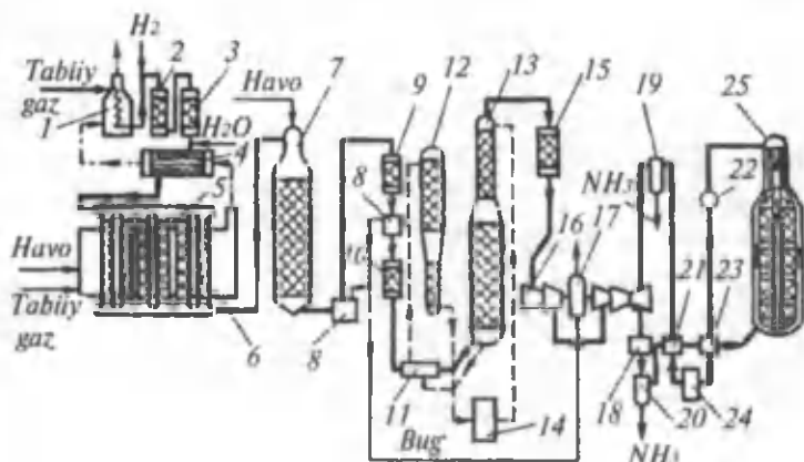
64- rasmda. Ammiak ishlab chiqarish sxemasi.
