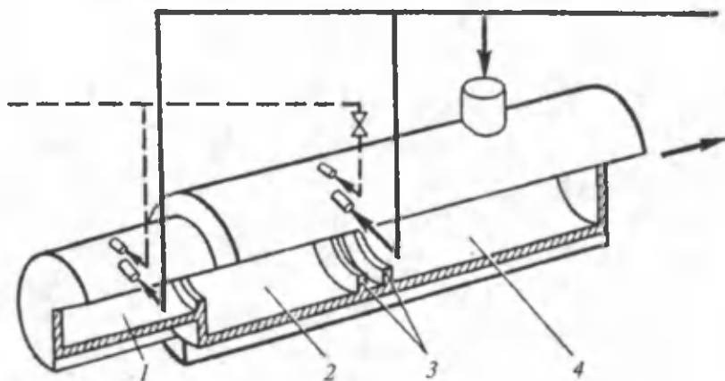
57- rasm. Oltingugurtni yoqish uchun ishlatiladigan siklon pechi.
