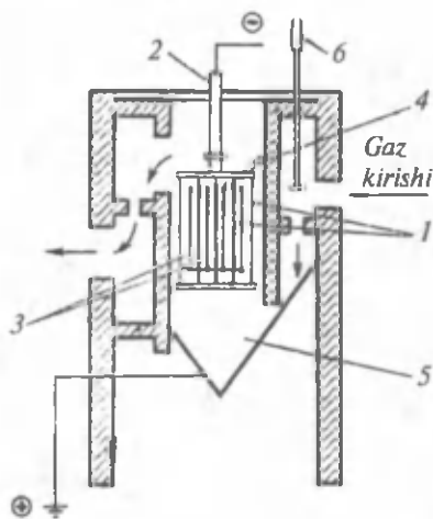
15- rasm. Plastinkasimon elektrofiltr.
