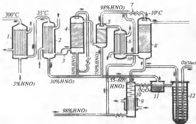
69- rasm. Konsentrlangan nitrat kislotasi sintezining sxemasi.
