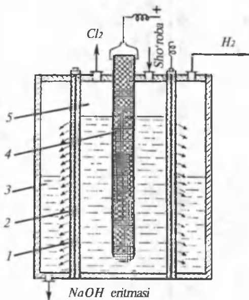
83- rasm. Filtrlovchi diafragmalı elektroliz vannasining sxemasi.
