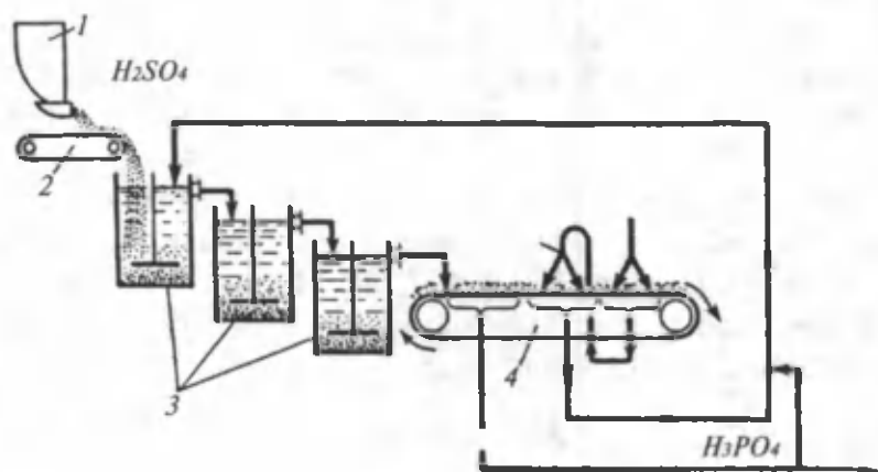
77- rasm. Ekstraksiya usuli bilan fosfat kislota ishlab chiqarish.
