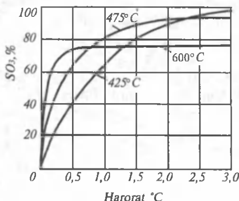
59- rasm. Turli haroratda va 0,1 MPa bosimda SO_2 oksidlanish darajasining vanadiyli katalizator bilan to'qnashuv vaqtiga bog'liqligi. ( SO_2 —7%, O_2 —11%, N_2 —82%).
