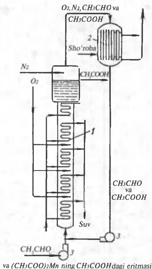
109- rasm. Sirka aldegidni oksidlab sirka kislota olish sxemasi.
