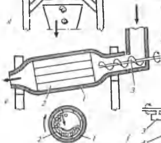
Sharlarning harakati sxemasi
