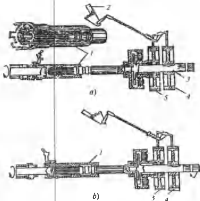
127-rasm. QOVning ishlash sxemasi:
