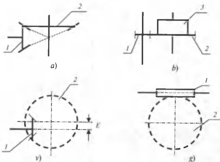
56-rasm. Yakkali bosh uzatmalarning sxemalari: a — konusli; b — silindrik; v — gipoid; g — chuvalchangsimon.
