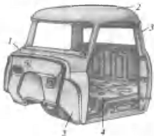
134-rasm. Ikki o'rinli yuk avtomobilining kabinasi: 1- yuqori panel; 2- tom; 3- orqa panel; 4- karkas; 5- yon panel.
