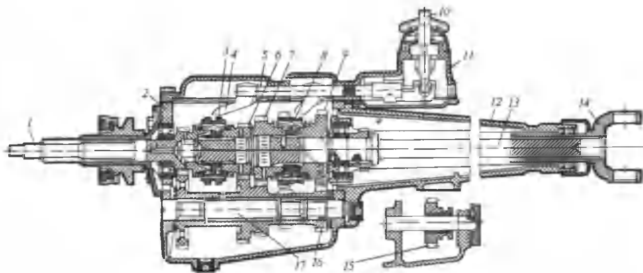
37-rasm. ГАЗ-3102 avtomobilining uzatmalar qutisi:
