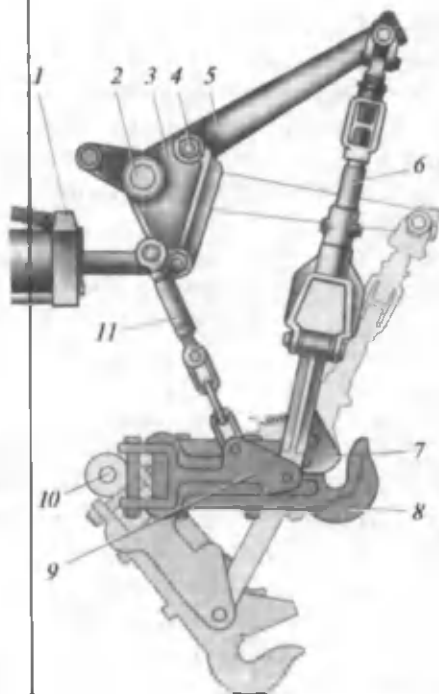
125-rasm. Hidrofitsirlangan ilmoq:
