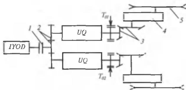
74-rasm. Zanjirli traktorning ikki bortli uzatma qutisiga ega bo'lgan kinematik sxemasi:
