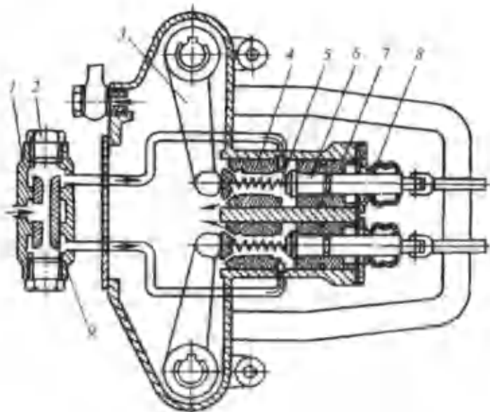
78-rasm. Bort friksionini boshqarish gidravlik servouzatmasining sxemasi:
