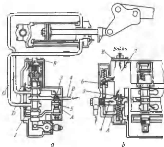
117-rasm. Gidrotaqsimlagichning neytral holatda ishlash sxemasi: a — o'tkazish klapanining ishlash sxemasi; b — saqlash klapanining ishlash sxemasi; 1 va 2- otvod (uzatish) kanallari; 3- o'tkazish klapani; 4- bosh kiritish kanali; 5- kalibrlangan teshik; 6- saqlash klapani; 7- to'kish bo'shlig'i.
