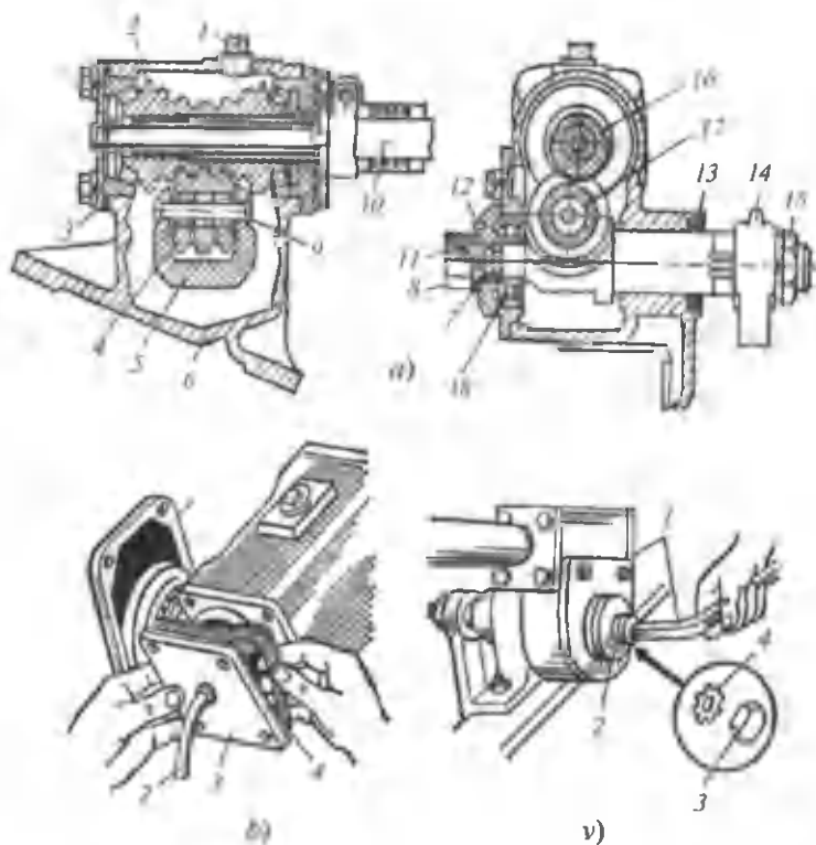
88-rasm. ГАЗ-53А avtomobilining rul mexanizmi va uni rostlash: a — tuzilishi: 1- moy quyish teshigining tiqimi (nazorat tiqimi); 2- chervyak; 3- qistirmalar; 4- uch o'rkachli rolik; 5- soshka vali; 6- quticha; 7- siljitmaydigan shayba; 8- gayka; 9, 17- uch o'rkachli rolikning o'qi; 10, 16- rul vali; 11- soshka valining rostlash vinti; 12- siljitmaydigan shtifti; 13- salnik; 14- rul soshkasi; 15- soshkani qotiradigan gayka, podshipnik; b — rul vali podshipnigini rostlash: 1- yon qopqog'i; 2- tovush signali simi; 3- pastki qopqog'i; 4- rostlash qistirmalari; v — chervyak rolik birikmasini rostlash: 1- maxsus kalitcha; 2- rostlash vinti; 3- vintning qalpoqsimon gaykasi (kontrgayka); 4- siljitmaydigan shayba.
