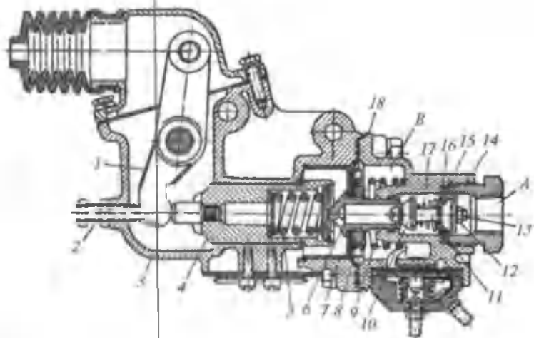
109-rasm. ЗИЛ-130 avtomobilining bir mexanizimli tormoz krani: A va B — kran bo'shliqlari; 1- yuritma richagi; 2- rostlash bolti; 3- kran qutichasi; 4- muvozanatlantiruvchi prujina stakani; 5- muvozanatlantiruvchi prujina; 6- chiqarish klapani uyasi; 7- diafragmaning yo'naltiruvchi stakani; 8- diafragma; 9- diafragmani dastlabki holatga qaytaruvchi prujina; 10- chiqarish klapani; 11- klapanlar orasidagi distansion quvursimon vtulka; 12- klapanlar o'zagi gaykasi; 13- klapanlar o'zagingin uchi; 14- kiritish klapani; 15- kiritish klapanining uyasi; 16- rostlash qistirmasi; 17- klapaning qaytarish prujinasi; 18- quticha qopqog'i.
