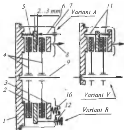
5-rasm. Ikki diskli doimiy qo'shilgan friksion ilashish muftasining prinsipial sxemasi:
