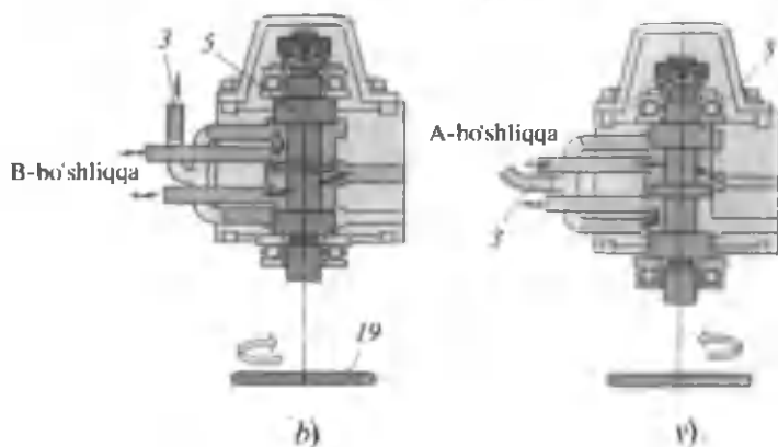
92-rasm. Hidrokuchaytirgichli rul boshqarmasining sxemasi: 1- porshen; 2- silindr; 3- ikki yekali sektor; 4- o'tkazish klapani; 5- zolotnik; 6- taqsimlagich; 7- shayba; 8- polzun; 9- saqlash klapani; 10- gidro- kuchaytirgichga moy haydash yo'li; 11 — chervyak; 12- soshka; 13- reyka; 14- prujina; 15- reyka tiragichi; 16- rul chambaragi; A, B — silindr bo'shliqlari; 17- differensialni blokirovkalash qismi; 18- eksentrik vtulka; 19- zolotnik gaykasi.
