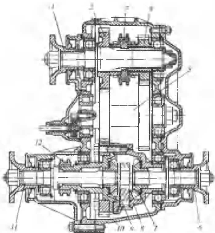
46-rasm. BA3-2121 «Нива» yengil avtomobilining taqsimlash qutisi: 1- yetakchi val; 2- sekinlashtiradigan uzatma shesternyasi; 3- uzatmalarni almashtiruvchi mufta; 4- yuqori uzatma shesternyasi; 5- oraliq val; 6- orqa ko'prik yuritmasining vali; 7- shesternya; 8- differensial korpusi; 9- satellitlar; 10- differensial shesternyasi; 11- oldingi ko'prik yuritmasining vali; 12- differensialni blokirovkalash muftasi.
