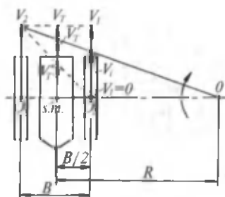
70-rasm. Zanjirli traktorning burilish sxemasini.
