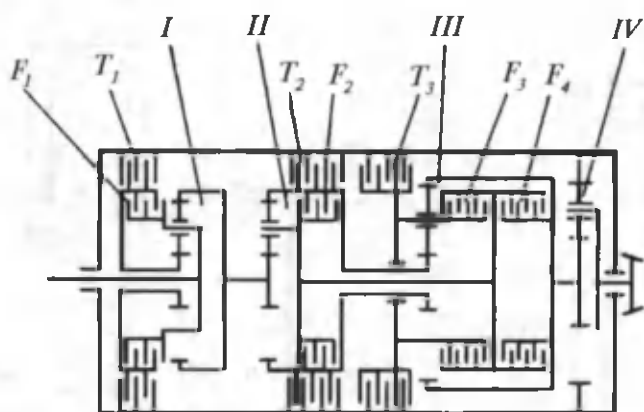
29-rasm. Tarkibli PUQ sxemasi.
