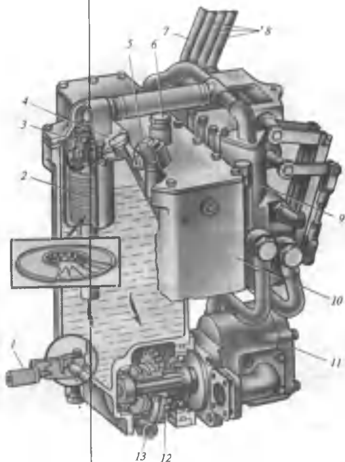
113-asm. MT3-80 traktorining moy baki:
