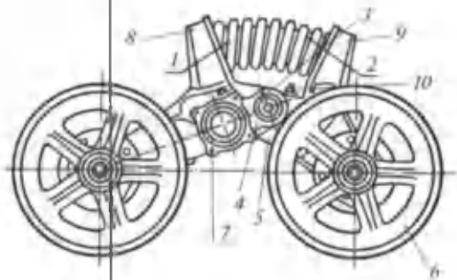
80-rasm. Zanjirli traktor elastik balansirli osmasining sxemasi:
