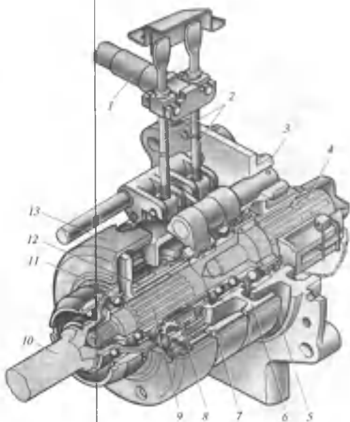
126-rasm. Planetar reduktorli QOV (MT3-80 traktori):
