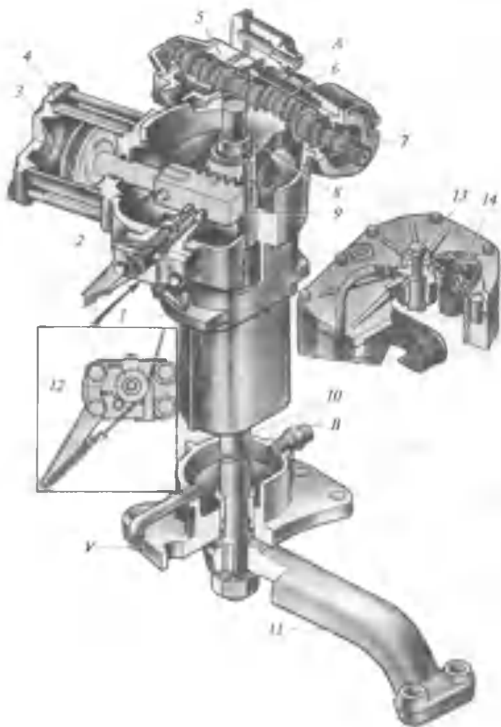
91-rasm. MT3-80 traktorining gidrokuchaytirgichli rul mexanizmi: 1- gidrokuchaytirgichli rul kolonkasi; 2- avtomatik blokirovka mexanizmi dastagi; 3- porshen; 4- silindr; 5- taqsimlagich; 6- chervyak; 7- eksentrik vtulka; 8- ikki yekali sektor; 9- reyka; 10- vertikal rul vali; 11- soshka; 12- turli filtr; 13- cheklash bolti; 14- quyish bo'g'zining qopqog'i. A — nasosga moy kirish yo'li; B — nasosdan moy chiqish yo'li; V — rul kolonkasidan moy to'kish yo'li.
