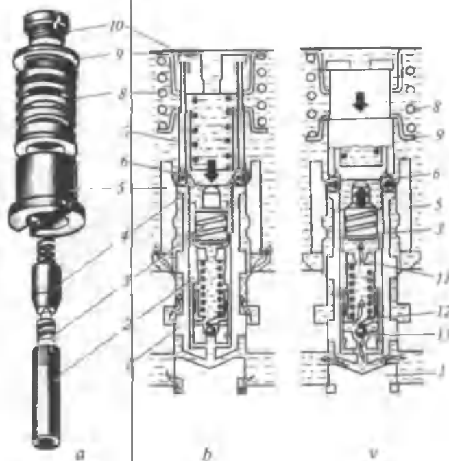
116-rasm. Zolotnikning fiksator qurilmasi va qaytarish mexanizmi:
