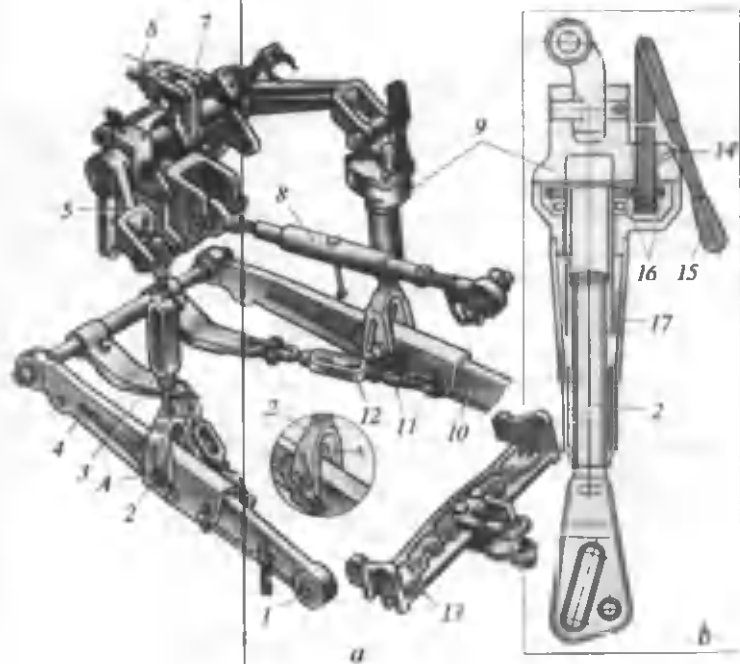
122-rasm. Uch nuqtali oʻrnatish mexanizmining sxemasi: a — tuzilishi; b — rostlanuvchi kashak; 1- sferik (sharli) sharnir; 2- kashak vilkasi; 3- chapki kashak; 4- boʻylama tortqining oldingi qismi; 5- boʻylama tortqining oʻqi; 6- silindr shtogi; 7- burish richagi; 8- markaziy tortqi; 9- oʻng kashak reduktor; 10- boʻylama tortqining orqa qismi; 11- cheklash zanjiri; 12- zanjirning taranglagichi; 13- tirkash qurilmasi; 14- moydon; 15- dasta; 16- shesternyalar; 17- kashak trubasi.
