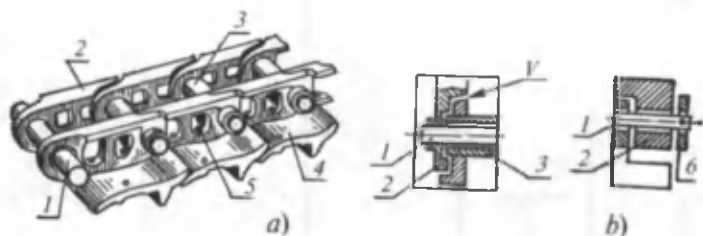
82-rasm. Himoyali va ochiq sharnirli zanjirlar:
