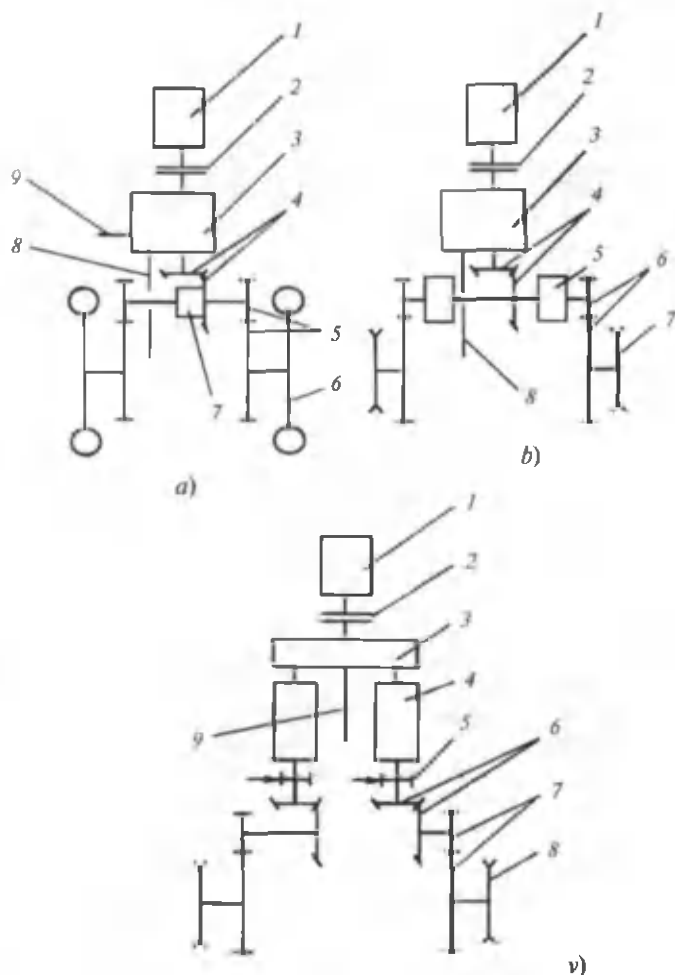
1- rasm. G'ildirakli va zanjirli traktorlarning prinsipial kinematik sxemalari: a) 1- dvigatel; 2- tishlashish muftasi; 3- uzatmalar qutisi; 4- markaziy uzatma; 5- oraliq uzatma; 6- yetakchi g'ildiraklar; 7- differensial; 8- orqa quvvat olish vali; 9- yon quvvat olish vali (QOV). b) 1- dvigatel; 2- tishlashish muftasi; 3- uzatmalar qutisi; 4- markaziy uzatma; 5- hurilish mexanizmlari; 6- oxirgi uzatma; 7- yetakchi yulduzcha; 8- orqa QOV. v) 1- dvigatel; 2- tishlashish muftasi; 3- taqsimlash qutisi; 4- uzatmalar qutilari; 5- tormozlash shkivi; 6- asosiy uzatmalar; 7- oxirgi uzatma; 8- yetakchi yulduzchalar.
