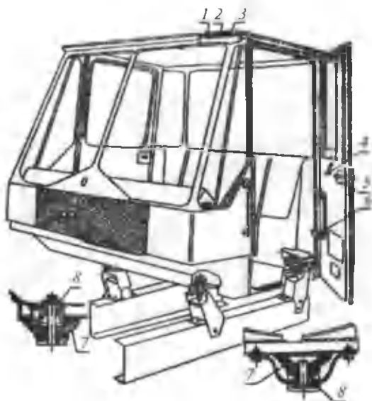
133-rasm. T-150K traktorining kabinasi: 1- mastika qatlami; 2- karton; 3- ekran; 4- oynani ko'tarish dastasi; 5- qulf; 6- oshiq-moshiq; 7- amortizator; 8- bufer.
