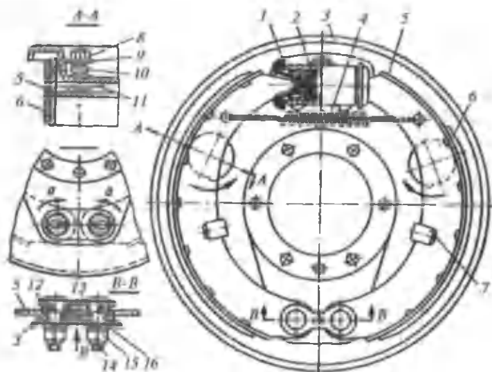
102-rasm. VAZ-53A avtomobilining oldingi g'ildirakka o'rnatilgan barabanli tormoz mexanizmi:
