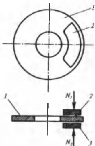
95-rasm. Avtomobillarda o'rnatiladigan diskli g'ildirak tormozi sxemasi: 1- aylanuvchi disk; 2, 3- friksion material qoplangan aylanmaydigan kolodkalar; N_1 , N_2 — diskni ikki tarfdan siquvchi kuchlar.
