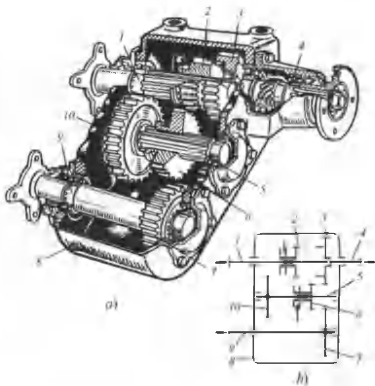
45-rasm. Sekinlashtiruvchi uzatmasi mavjud bo'lgan taqsimlash qutisi: a — tuzilish sxemasi; b — kinematik sxemasi; 1- yetakchi val; 2- qo'z-g'aluvchan shesternya; 3- yetaklanuvchi val bilan birga ishlangan shesternya; 4- yetaklanuvchi val; 5- oraliq val; 6- oldingi ko'prikn ulovchi shesternya; 7- shesternya; 8- taqsimlash qutisining korpusi; 9- oldingi ko'prikn yuritmasining vali; 10- sekinlashtiruvchi uzatma shesternyasi.
