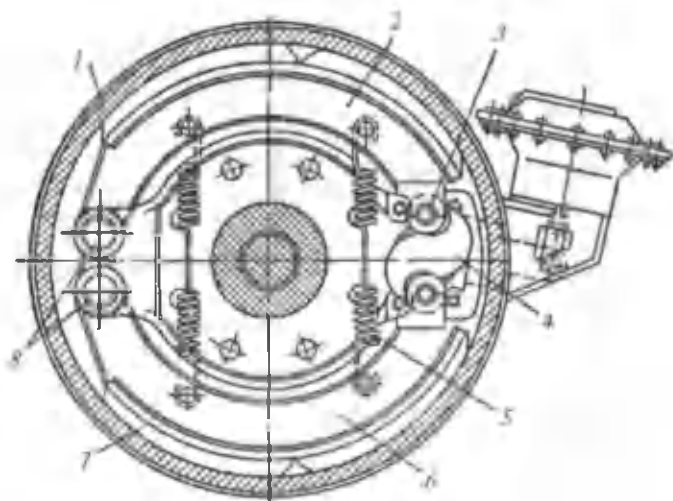
110-rasm. ЗИЛ-130 avtomobilining orqa g'ildirak tormozi: 1- tormoz barabani; 2, 6- tormoz kolodkalari; 3- kolodka roligi; 4- keruvchi moslama; 5- kolodkalarni bir-biriga tortuvchi prujina; 7- kolodkaning friksion ustqoymasi; 8- kolodkaning tayanch harmog'i.
