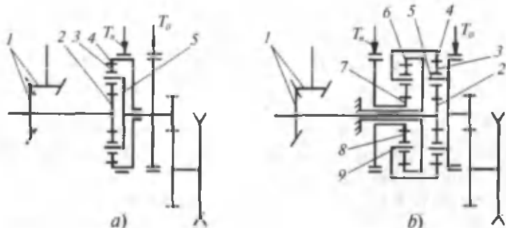
72-rasm. Bir pog'onali planetar burilish mexanizmi sxemalari: 1- markaziy uzatma; 2- quyoshsimon shesternyasi; 3- satellit; 4- episiklik shesternya; 5- vodilo; 6, 7, 8 va 9- episiklik shesternya, quyoshsimon shesternya, satellit va qo'shimcha planetar qatorining vodilosi; T_p - burilish tormozi; T_0 - to'xtatish tormozi.
