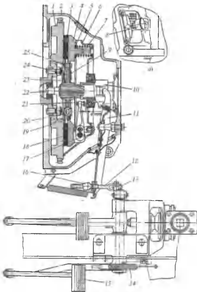
10-rasm. ГАЗ-53А avtomobilining ilashish muftasi va yuritmasi:
