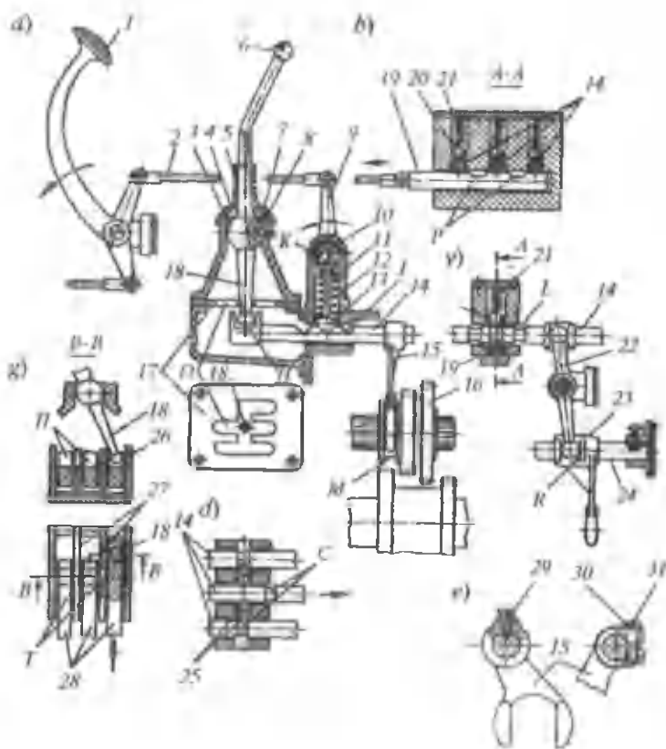
38-rasm. UQni boshqarish mexanizmlarining prinsipial sxemalari.
