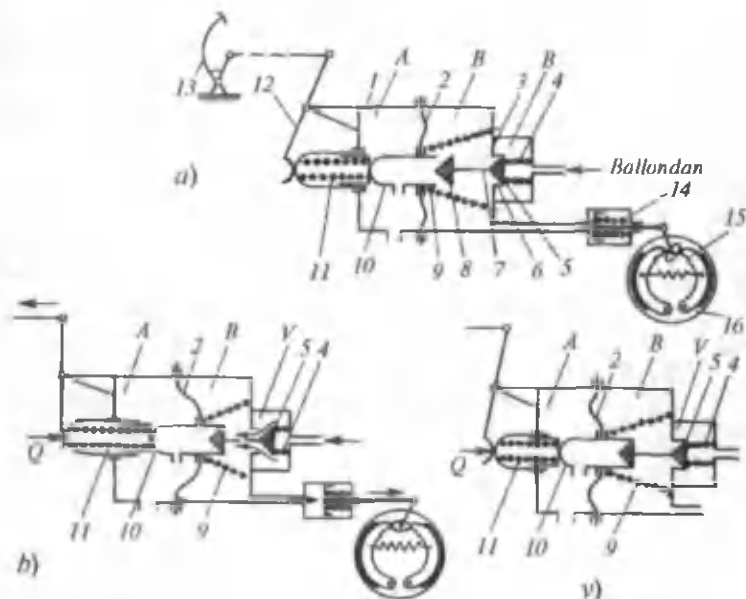
99-rasm. To'g'ri harakatlantiruvchi diafragmali moslagich mexanizmining sxemasi:
