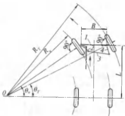
86-rasm. To'rt g'ildirakli mashinaning burilish sxemasi va rul trapetsiyasi: 1- mashinaning oldingi o'qi; 2, 4- burilish sapfalarining richaglari; 3- ko'ndalang rul torkisi; 1, 2, 3, 4- rul trapetsiyasi; 5- bo'ylama rul torkisi.
