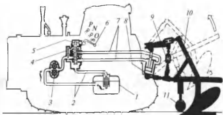
112-rasm. Traktor o'rnatma gidrotizimining sxemasi:
