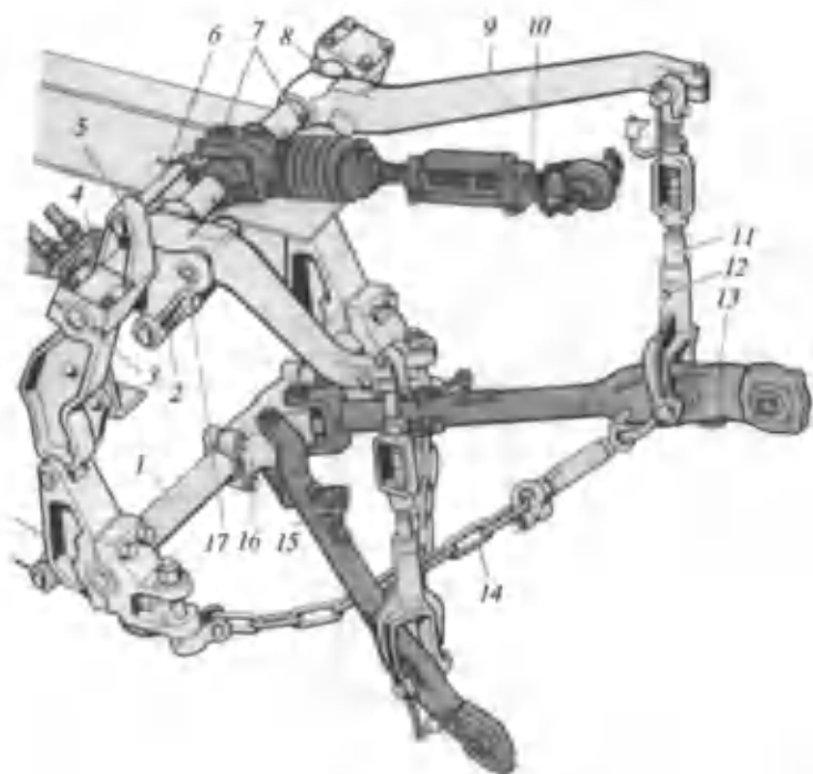
121-rasm. T-150K traktorining ikki nuqtali o'rnatish mexanizmi: 1- pastki o'q; 2- shtokning burish richagi; 3- yuqorigi o'q; 4- kuch silindri; 5- tirgak richagi; 6- blokirovkalash barmog'i; 7- moydon; 8- yuqorigi o'q; 9- ko'tarish richagi; 10- markaziy tortqi; 11- kashak; 12- stoporlash barmog'i; 13- pastki tortqi; 14- cheklash zanjiri; 15- teleskopik ulash barmog'i; 16- markaziy kallak; 17- teshik.
