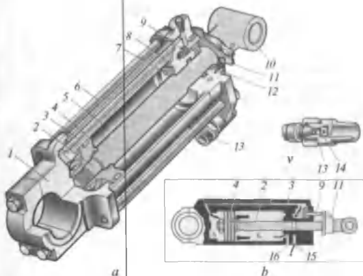
120-rasm. Gidrosilindr:
