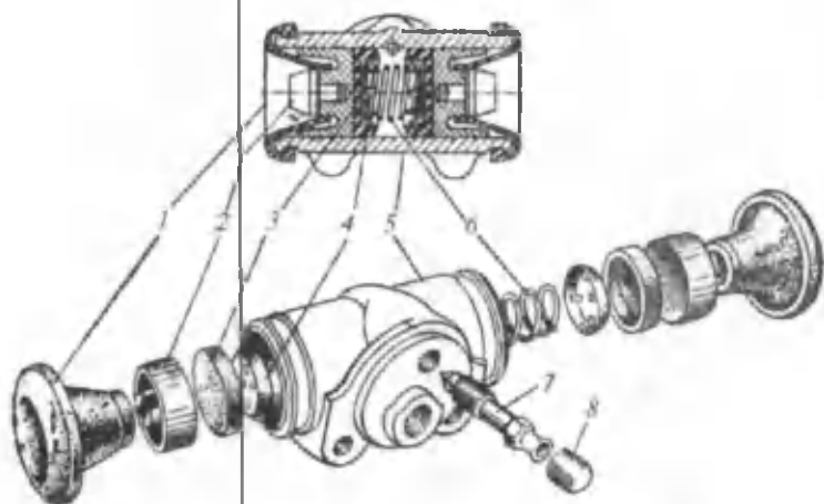
103-rasm. G'ildirak tormoz silindri:
