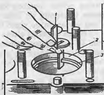
58-rasm. Porshen halqasini tutashish joyidagi tirqish o'lchamini aniqlash: 1-shup; 2-silindr ichki yuzasi; 3-porshen halqasi
