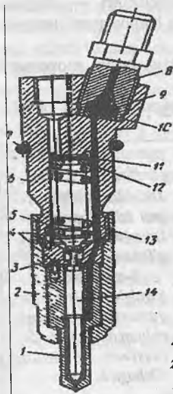
73-rasm. «KamAZ-740» dvigatelining forsunkasi
