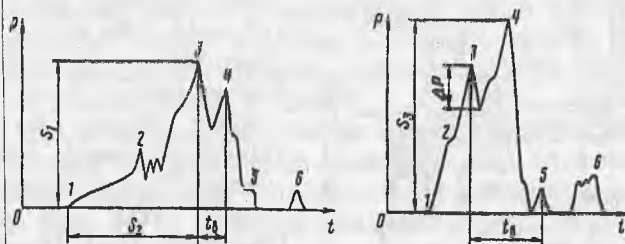
70-rasm. Forsunka shtutserida hosil bo'lgan bosim ossillogrammasi:
