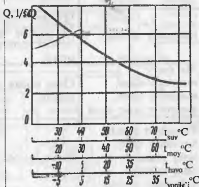
124-rasm. Dvigatelni qizdirish uchun sarfladigan issiqlik sarfining boshlang'ich haroratga bog'liqligi.
