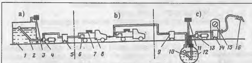
118-rasm. Diyezol yonilg'isini tashib kelish, saqlash va tarqatishda tozalash shakli:
