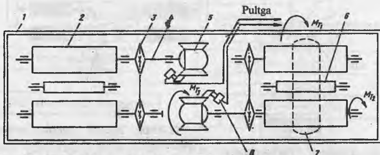
33-rasm. Kuchlar orqali ishlovchi rolikli tormoz jihozi shakli:
