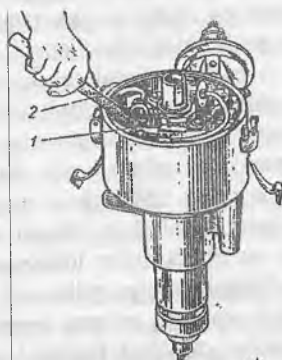
68-rasm. Uzgıch kontaktlarını sozlash(a) va tozalash(b): 1-kontaktlar, 2-abrazıv plastana.
