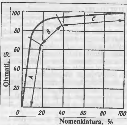
112-rasm. Detal va materiallarning nomenklatura va qiymati bo'yicha bir-biriga bog'liqlik grafiqi.
