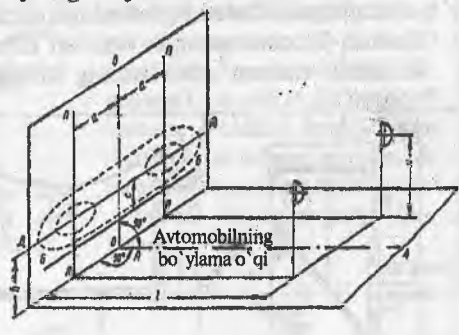
93-rasm. «Evropacha» assimetrik yorug'lik faralarini tekshirish.
