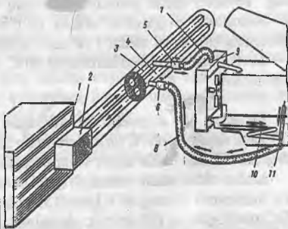
129-rasm. Avtomobil dvigatelini issiq suv yordamida o'tildirishdan avvalgi bir zumdagi isitishning prinsipial shakli:
