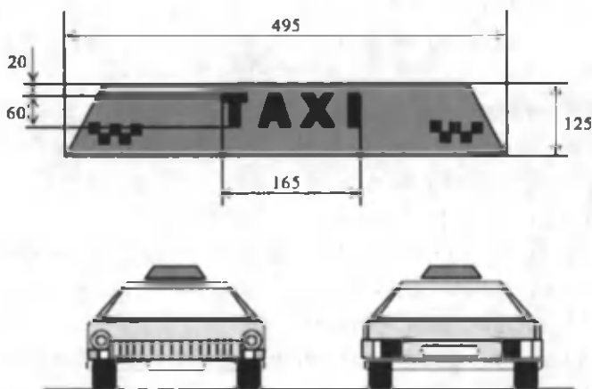
4.1.-rasm. «TAXI» tanish belgisining tasviri va o'lchamlari (mm)
