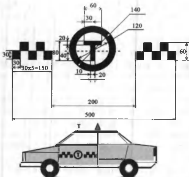
4.2.-rasm.Yo'nalishsiz taksilarning oldingi eshiklariga chiziladigan qora kvadratlar va «T» harfidan iborat kompozitsiyaning tasviri va o'lchamlari (mm).
