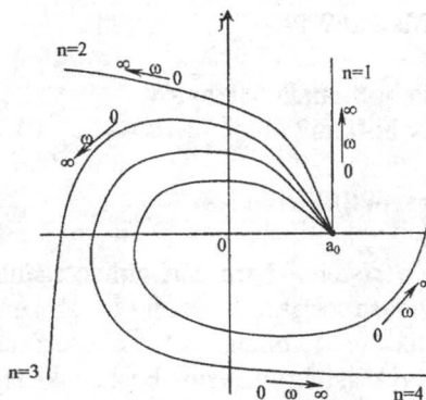
5.3-rasm. Barqaror sistemalar godograflari
