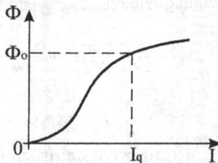
2.3-rasm. Magnitlanish grafigi.
