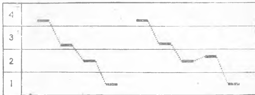
Расми 39. Тонотрамаи ҷумлаҳои Гиред ўро! Хонед мактубро.
