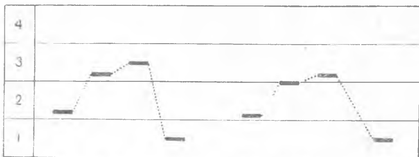
Расми 32. Тонограмман ҷумлаҳои Бобо омад. Баҳор гузашт.
