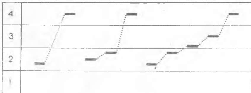
Расми 41. Тоногограммаи ҷумлаҳои Хомӯш! Оҳиста! Як пиёла чой!
