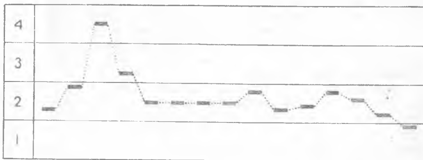
Расми 37. Тонограммаи ҷумлаи Ту аз кай боз дар Тоҷикистон зиндагӣ мекуӣ?
