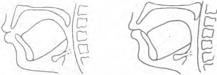
Расми 15. Рентгенограммаҳои фонемаҳои б (1) ва п (2).
