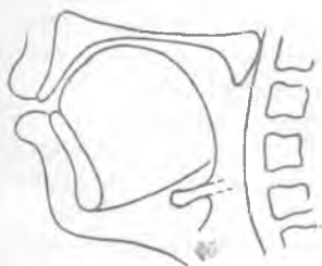
Расми 26. Рентгенограммаҳои ҳамсадоҳои г (1) ва к (2).
