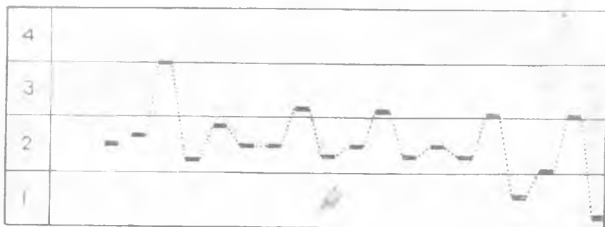
Расми 43. Тонограмми чумлаи Гулсара духтари мешчашм, мушқинмӯ, қадбаланд, сафедруӣ буд.
