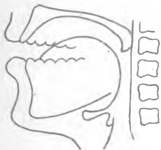
Расми 11. Рентгенограм- маи садоноки у.
