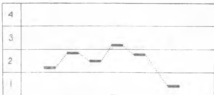
Расми 33. Тонограммаи ҷумлаи Бобо бобо дорад.
