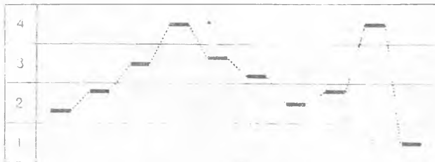
Расми 38. Тонограммаи ҷумлаи Меҳмонон имрӯз меоянд ё фардо?
