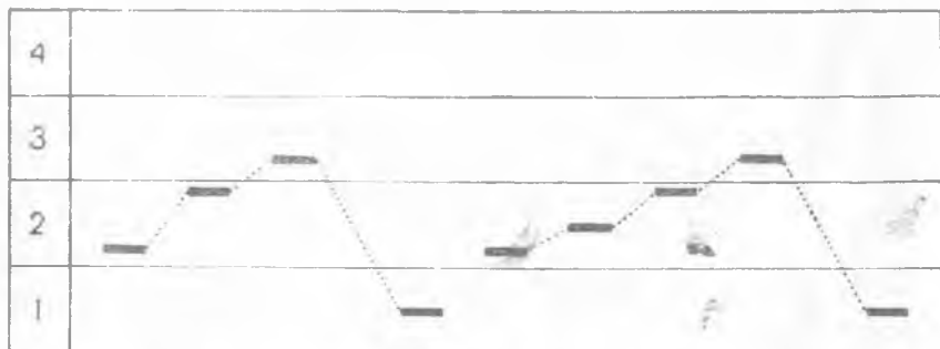
Расми 34. Тонотраммаҳои ҷумлаҳои Сардор омад. Барон гузашт.
