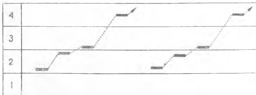
Расми 35. Тонотраммаҳои ҷумлаҳои Сардор омад? Маҷлис сар шуд.
