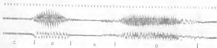
Расми 3. Осциллограммаи калимаи сақо.
