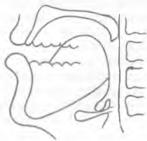
Расми 14. Рентгенограмман садонокӣ о.
