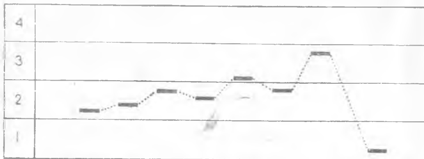
Расми 40. Тонोगраммаи ҷумлаи Тараддудатро дидан гир!
