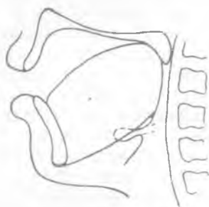
Расми 27. Рентгенограммаи ҳамсадои қ.
