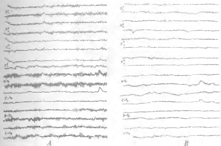
24-rasm. A — asabi tinch odamning elektroensefalogrammasi. EEGda bir maromli \alpha - to'liqlar ko'zga tashlanadi; B — asabiylashgan odamning elektroensefalogrammasi. Unda \alpha - to'liqlar yo'q, miyaning barcha nuqtalari bo'ylab yuqori chastotali, past amplitudali \beta - to'liqlar ro'yxatga olingan (Z.R. Ibodullayev kuzatuv, 2004)
