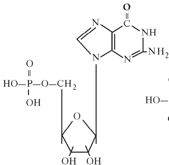
Guanil kislota yoki guanilmonofosfat (GMF)
