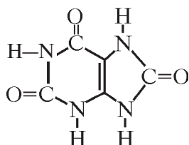
siydik kislota (2, 6, 7-trioksiipurin)
