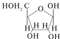
\beta -D-ribofuranosa
