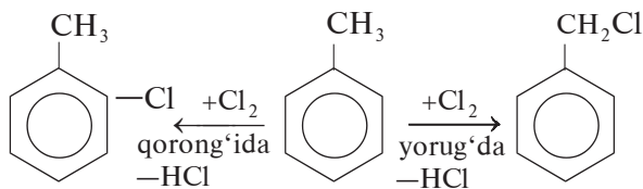
o - xlortoluol
