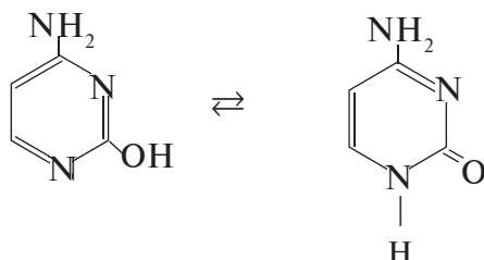
2-oksi-4-aminopirimidin (sitozin)
