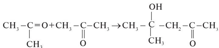
diaseton spirt (4-oksi-4 metil pentanon-2)
