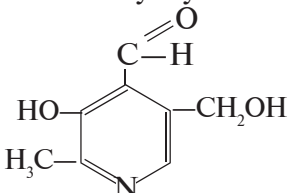
piridoksal
