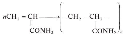
poliakrilamid
