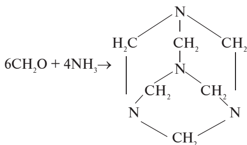
urotropin (geksametilen tetramin)
