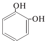
ikki atomli
