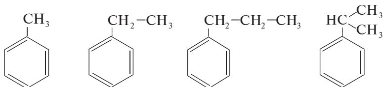
metilbenzol
