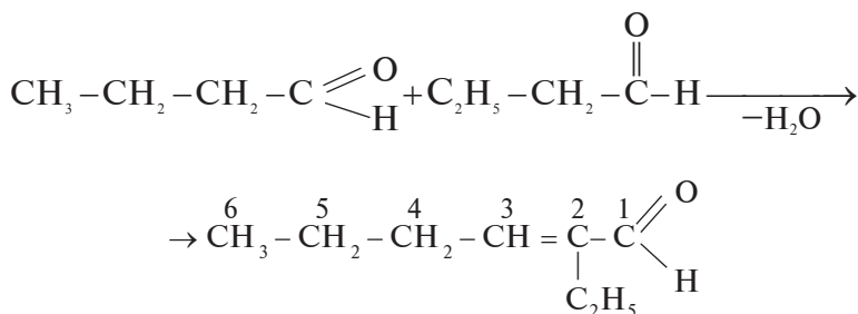
2-etilgeksen-2-al
