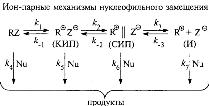
Схема 9.2
