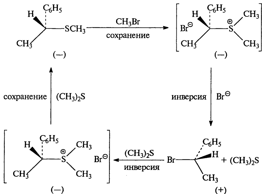
Схема 9.1
