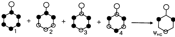
Рис. 13.6. \pi -МО молекулы C_6H_5X
