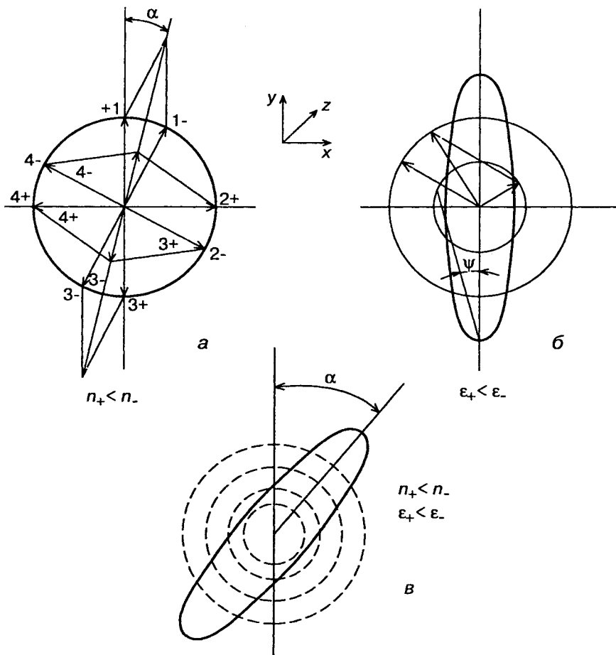
Рис. 8.2. а — Взаимодействие сдвинутых по фазе компонент равной амплитуды; б — взаимодействие находящихся в фазе компонент разной амплитуды; в — суммарный результат сдвига по фазе. Точки 1, 2, 3, 4 соответствуют точкам на рис. 8.1, б и в. Знак «плюс» для правого луча, знак «минус» для левого «отстающего» и более сильно поглощаемого луча
