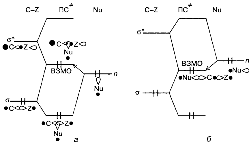
Рис. 9.2. Диаграмма возмущения граничных орбиталей в S_N2 -реакции при фронтальной (а) и тыловой (б) атаке нуклеофила (Nu) на связь C–Z. PC^\ddagger — переходное состояние
