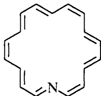
аза-[18]-аннулен
