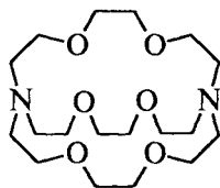
криптанд[2,2,2]
