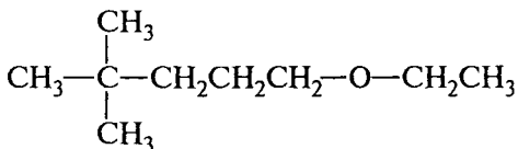
1-этоксн-4,4-днметнлпнтан
