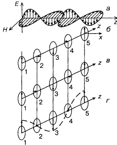
Рис. 8.1. Плоско (линейно) поляризованный световой луч ( a ), правый ( b ) и левый ( c ) циркулярно поляризованные лучи (показаны только векторы электрического поля). z — Результат взаимодействия электрических векторов лучей ( b ) и ( c ), находящихся в фазе
