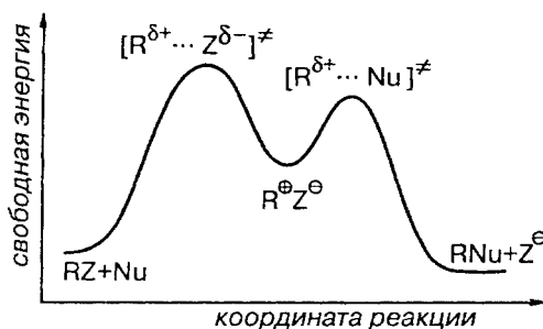
Рис. 9.6. Первая стадия ионизации RZ
