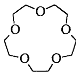
15-краун-5
