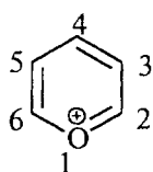
катион пирилия
