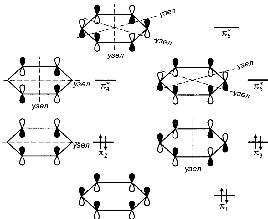
Рис. 12.1. Симметрия и узловое свойства молекулярных орбиталей бензола
