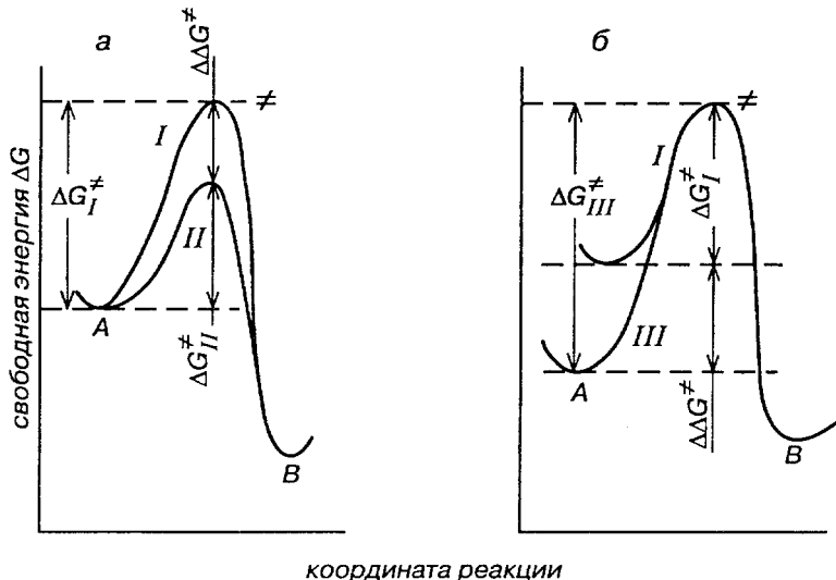
Рис. 9.5. Энергетические профили реакций: а — с несольватированным ( I ) и сольватированным ( II ) переходным состоянием; б — с несольватированными ( I ) и сольватированными ( III ) исходными реагентами.
