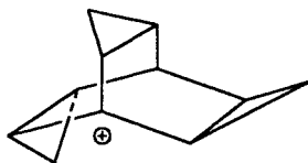
1-трис-гомобаррелильный катион
