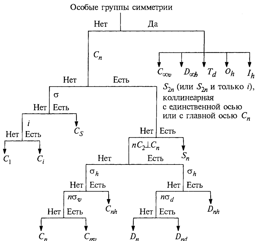
Схема 8.1
