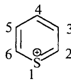
катион тиопирилия
