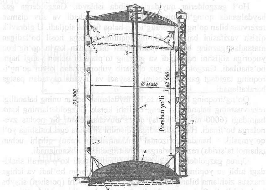
9.3-rasm. Hajmi 100000 m 3 bo'lgan suyuqlikli zatvorli quruq gazgolder: 1-yopilmasi; 2-shaybaning yuqori holati (porshen); 3-chiqish narvoni; 4-ko'taruvchi panjara; 5-gazgolder devori; 6-shayba; 7-tashqi ko'targich; 8-gaz uzatma.
