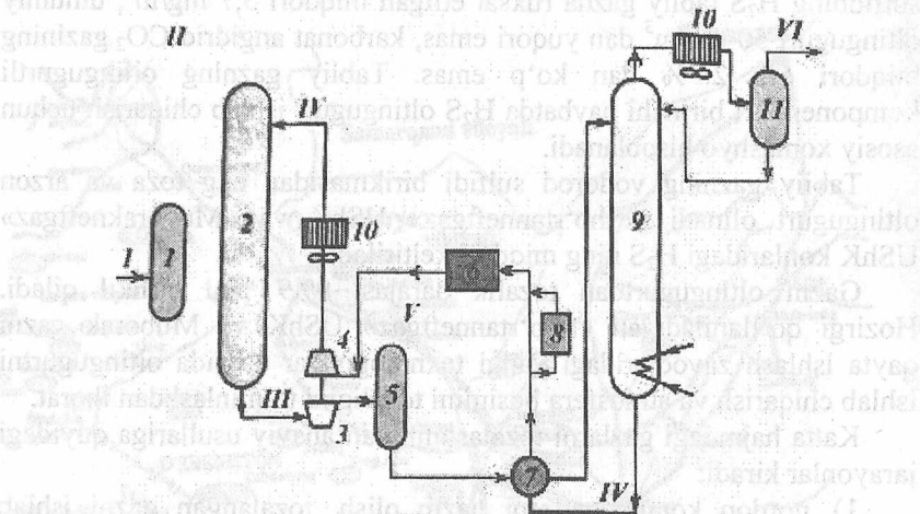
7.6-rasm. Kimyoviy absorbsiya usulida tabiiy gazni tozalash qurilmasining sxemasi:
