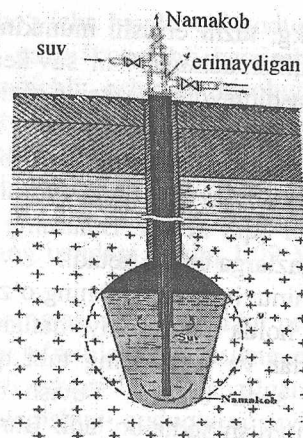
9.12- rasm. Tosh tuzli yotqiziqlarda qurilgan yer osti sig'imining texnologik sxemasi:
