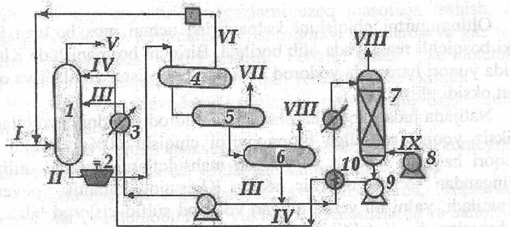
7.7-rasm. Fizik absorbsiya usulida gazni quritish qurilmasining sxemasi:
