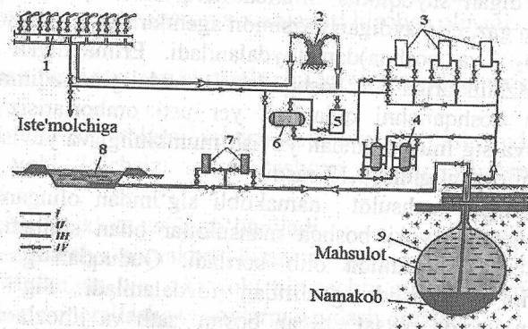
9.13-rasm. Tosh tuzni yotqiziqlardagi suyultirilgan gazlarning yer osti omborlarini ishlatish sxemasi:
