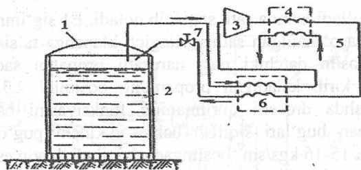
9.10-rasm. Suyultirilgan gazni rezervuarda past bosimli rejimda ushlab turishning prinsipial sxemasi: 1-rezervuar; 2-suyultirilgan gaz; 3-kompressor; 4-issiqlik almashtirgich-kondensator; 5-sovutishga yo'naltirilgan suv; 6-issiqlik almashtirgich; 7-drossellash jo'mragi.
