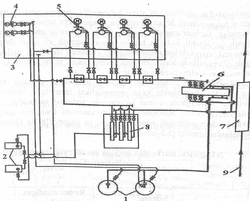
5.2-rasm. Oraliq nasos stansiyasining texnologik sxemasi:
