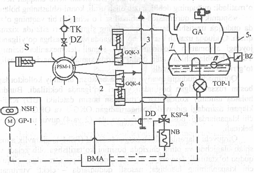
4.8-rasm. «Sputnik-A» avtomatik guruhli o'lov qurilmasining prinsipial sxemasi:
