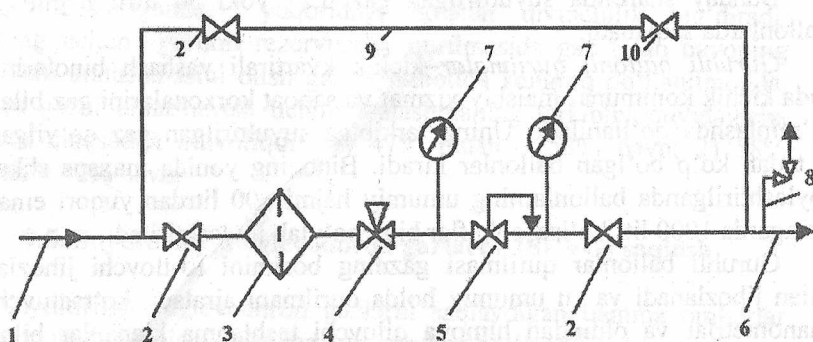
9.7- rasm. Gazni rostlash punktining (GRP) texnologik sxemasi:
