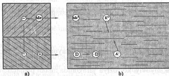
10.8-rasm. Elektrokimyoviy korroziyon jarayon sxemasi.
