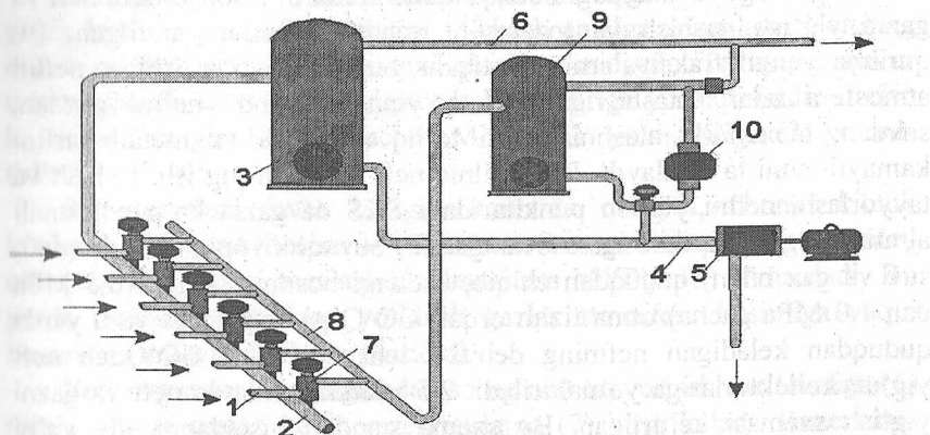
2.4 - rasm. Guruhli o'lchash qurilmasida debitni o'lchashning prinsipial sxemasi:
