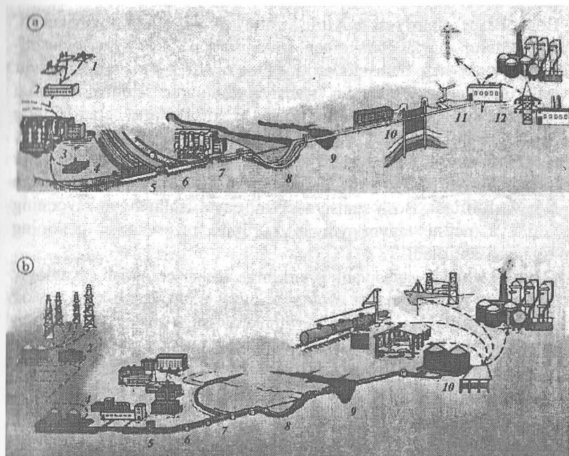
5.1-rasm. Magistral gaz uzatmalarining va neft uzatmalarining sxemasi:
