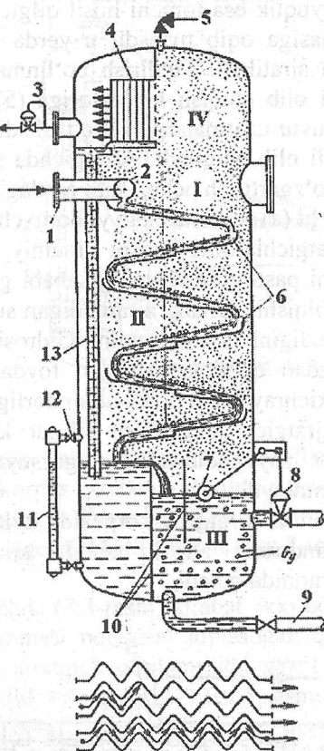
7.1-rasm. Tik ajratgich qurilmasi:
