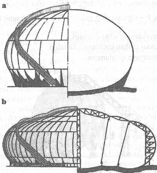
5.4-rasm. Tomchi ko'rinishli rezervuarlar: a-silliq; b-ko'p torsli.
