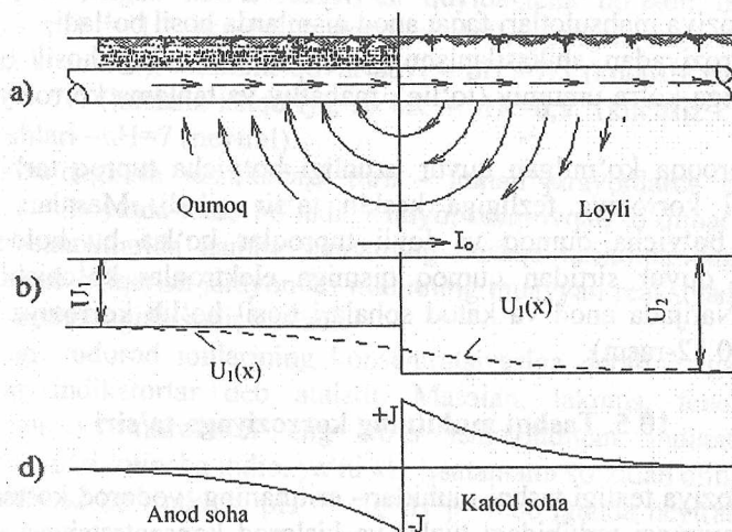
10.12-rasm. Yer osti quvurida korrozion makrojuftlikning hosil bo'lishi. a – quvur sxemasi; b – quvur-tuproq potentsiallar farqining o'zgarishi; d – quvur bo'ylab korroziya toki zichligining o'zgarishi.
