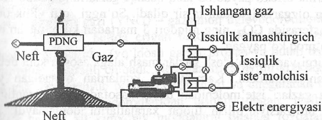
3.2 - rasm. Yoʻldosh neft gazini gaz elektr stansiyasida utilizatsiya qilish.
