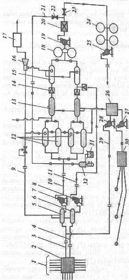
4.7-rasm. Neft, gaz va suvni yuqori bosimli gernetiklangan va avtomatlashtirilgan yig'ishning sxemasi: 1-otma chiziq; 2-avtomatik guruhli o'lchash qurilmasi (AGO'Q); 3,4-yig'ish kollektorlari; 5-suvlangan neft uchun ajratgich; 6-toza neft uchun ajratgich; 7,8-mahsulot uzatuvchi nasoslar; 9-gaz uzatma; 10,11-NTQga beruvchi quvur uzatmalar; 12-ajratgichlar-qizdirgichlar; 13-tindirgich; 14-shtuser; 15-ajratgich; 16-ejektor; 17-gazni qayta ishllovchi zavod (GQIZ); 18-gernetiklangan rezervuar; 19-nasos; 20-ATO'Q (Rubin 2); 21-neft chizig'i; 22,23-zulfin; 24-tovar rezervuari; 25,27,28-nasoslar; 26-suvni tozalash qurilmasi (STQ); 27,28-nasos; 29-suv uzatmasi; 30-BSHNS; 31-kanalizatsiya; 32-suvsizlantirgich va tuzsizlantirgich.
