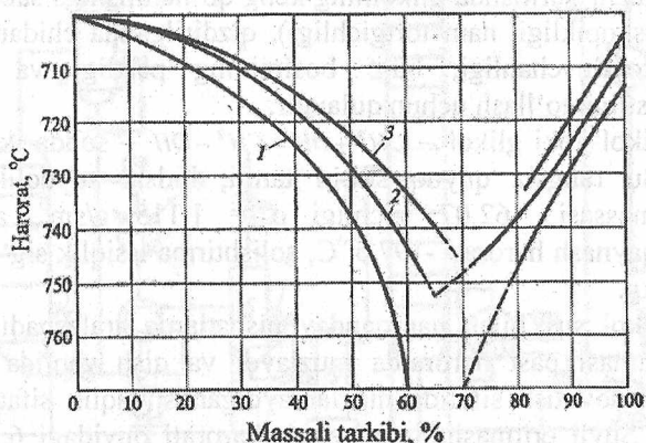
6.2-rasm. Suvli eritmalarini muzlash haroratini tarkibga bog'liqligi: 1 – etilenglikol; 2 – dietilenglikol; 3- trietilenglikol.
