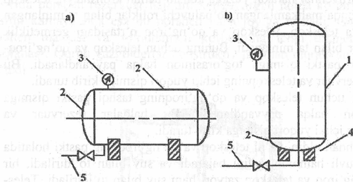
9.4-rasm. Yuqori bosimli silindrik gazgolderlar : a) yotiq; b) tik.
