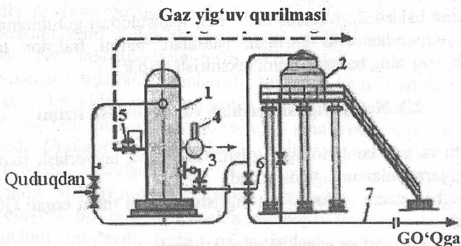
2.2-rasm. Neftni yig'ishda o'zi oqar tizimining individual o'lchov qurilma sxemasi:
