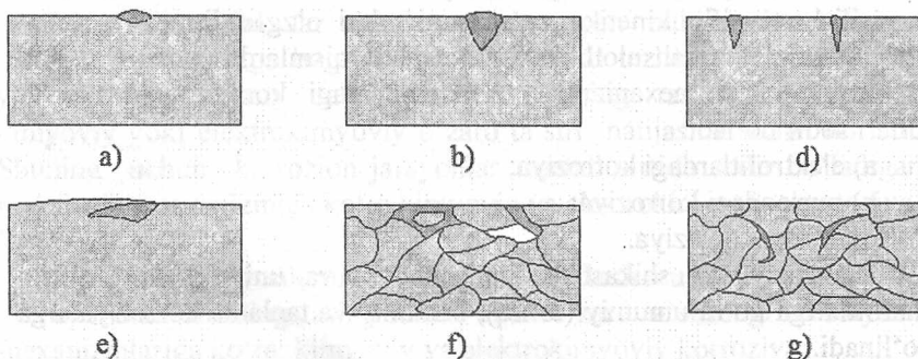
10.2-rasm. Mahalliy korroziya ko'rinishlari.
