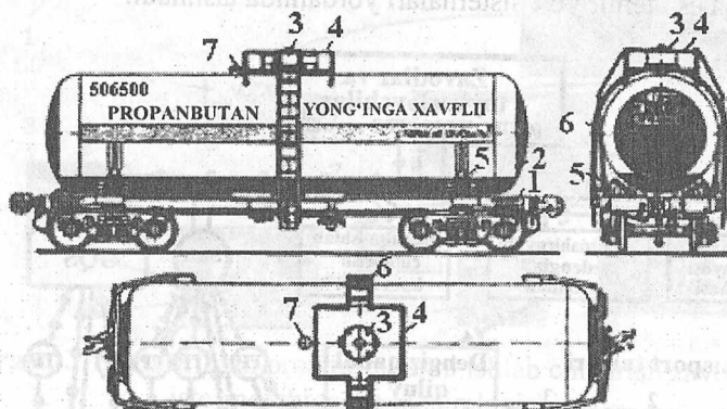
8.3-rasm. Suyultirilgan neft gazini tashish uchun temir yo'l vagon - sisternasi:
