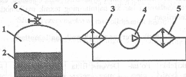
9.9- rasm. Rezervuarda suyultirilgan gazni past haroratli rejimda ushlab turish sxemasi: 1-rezervuar; 2-suyultirilgan gaz; 3-issiqlik almashtirgich; 4-kompressor; 5-sovutgich; 6-drosellash ventili.
