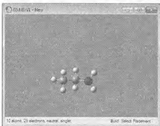
7-rasm. Etilamin molekulası.
