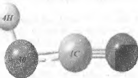
49-rasm. Sianit kislota molekulasining geometrik strukturasi.
