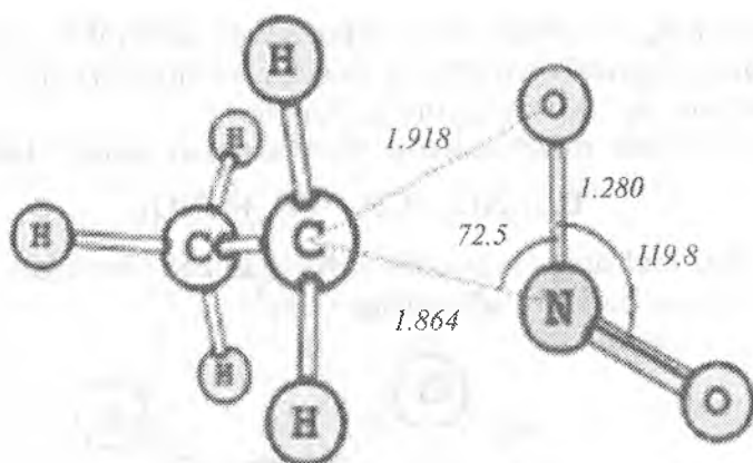
42-rasm. Nitrometan molekulasida nitro-nitritli qaytaguruhlanish reaksiyasida o'tish holati.
