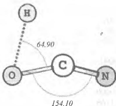
52-rasm. QST3.gjf fayli uchun o'tish holatining geometrik strukturasi.
