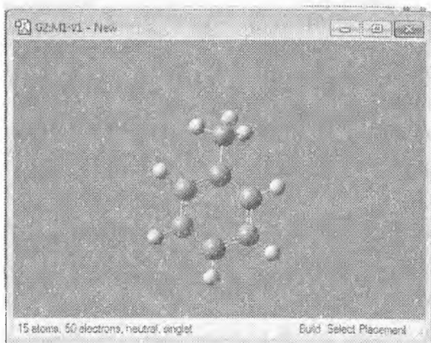
11-rasm. Metilbenzol molekulasiga.
