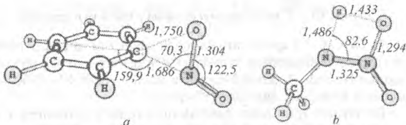
18-rasm. Reaksiyalarning o'tish holati reaksiyalari: a) nitrobenzolda nitro-nitritli qayta guruhlanib b) metilnitroamin atsi-formasining hosil bo'lishi.
