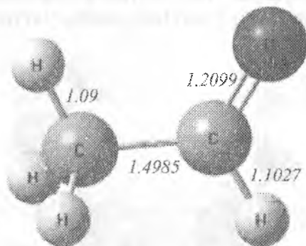
46-rasm. Sirka aldegidli molekulasining geometrik strukturasi.
