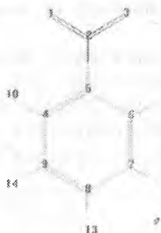
Atomlari raqamlangan molekulaning umumiy ko'rinishi
