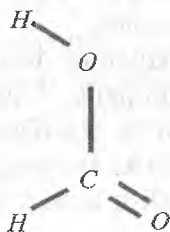
8-rasm. Chumoli kislota molekulasiining strukturasi.
