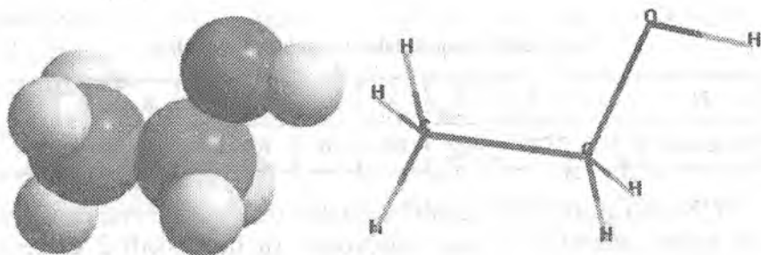
6-rasm. Etanol molekulasini modellari.
