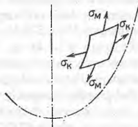
91-rasm. Halqali va meridianal kuchlanishlar ta'sirining sxemasi.
