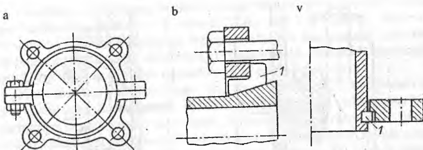
100-rasm. Flanelarni ajraladigan turlari: a – bo‘laklarga bo‘linadigan; b – halqaga bo‘linadigan; v – joylanadigan halqa.
