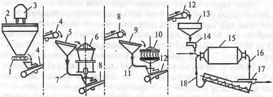
23-rasm. Maydalashning prinsipl texnologik sxemasi:
