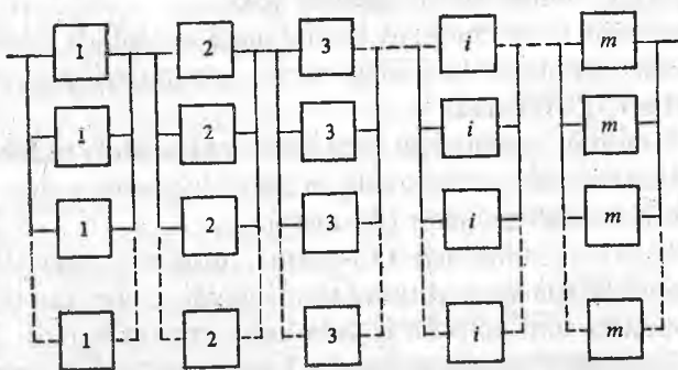
86-rasm. Alohida zaxiralash blok-sxemasi (doimiy ulangan zaxira bilan).
