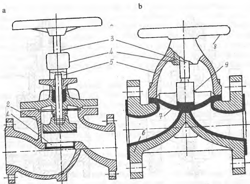
65-rasm. Flanetsli (a) va diafragmali (b) jo'mraklar: 1 — egar; 2 — zolotnik; 3 — shpindel; 4 — vtulka; 5 — skoba; 6 — korpus; 7 — membrana; 8 — maxovik; 9 — krestovina.
