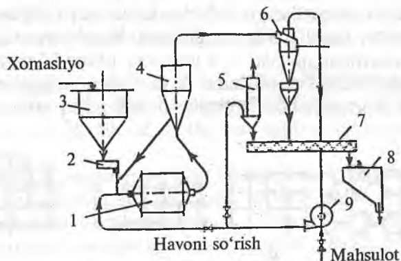
24-rasm. Maydalagichning quruq sxemasi:
