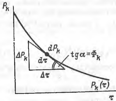
112-rasm. R_k bo'lib turish ehtimollik vaqtining qiymati va F_k ehtimollik taqsimlanish zichligi o'rtasidagi nisbat
