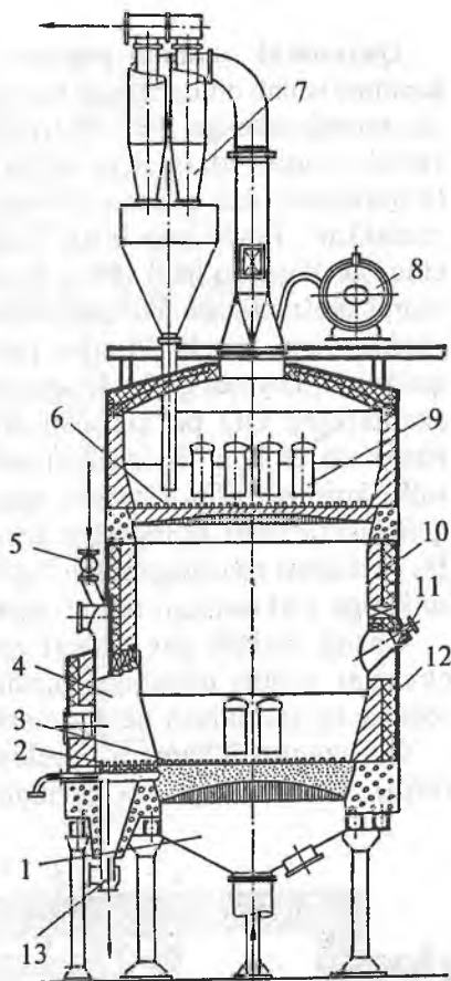
37-rasm. Kolchedonni kuydirish uchun DKSM pechi: 1 — dam berish bo'limasi; 2 — dam berish ta'sirida to'ng'ariladigan panjara; 3 — to'ng'arilmaydigan panjara; 4 — yuklash bo'limasi; 5 — retur ta'minlagichi; 6 — bo'lish panjarasi; 7 — qaytarish siklonlari; 8 — qozon barabani; 9 — sovitish elementlari; 10 — qoplama; 11 — kuzatish darchasi; 12 — pech g'ilofi; 13 — bo'shatish zatvori (eshigi).
