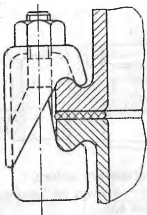
101-rasm. Skobalar bilan tortiladigan flanesli birikma
