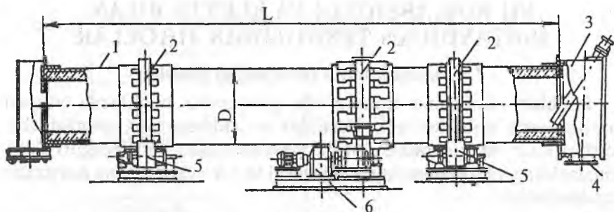
34-rasm. Ikki tayanchli suriladigan kallakli aylanma pech: 1 – korpus; 2 – belbogʻ (bandaj); 3 – suriladigan kallak; 4 – patrubok; 5 – roliklar; 6 – reduktorli elektruyitgich.
