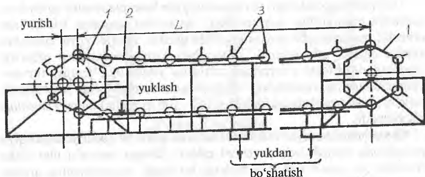
48-rasm. Qovurg'ali konveyer:
