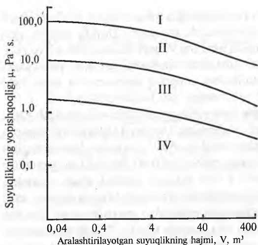
6-rasm. Turli xil aralashtirgichlarning qo'llanilish oralig'i (diapazoni):
