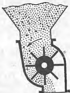
73-rasm. Bo'lmali ta'minlagich.
