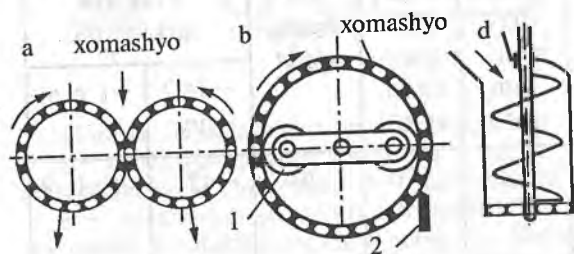
32-rasm. Ekstruzion tipdagi donalagichlar:
