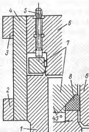
97-rasm. Siquvchi vintlar va ajratgich muftalar hilan majburiy zichlovchi plastik trapetsiyasimon obturatorli boltli zatvor.
