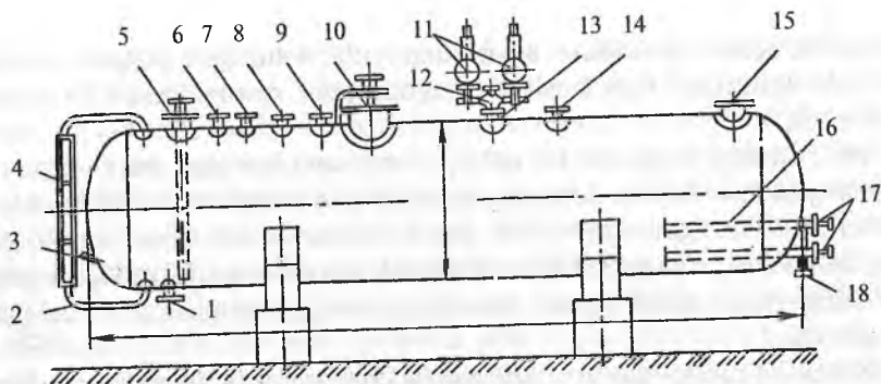
80-rasm. Suyuq ammiak uchun rezervuar jihozlarning sxemasi:
