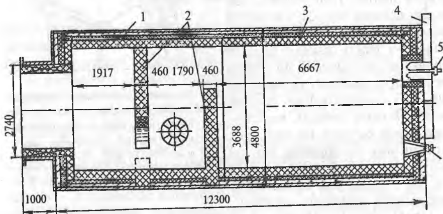
38-rasm. Suyultirilgan oltingugurtning yondirish uchun kamerali pech: 1 — korpus; 2 — teshiklar o'yilgan to'siqlar; 3 — qoplama; 4 — havo kirishi uchun g'ilof; 5 — oltingugurt uchun purkagich; 6 — mazut purkagichi.
