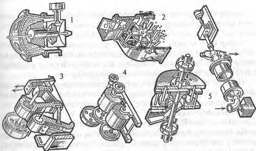
18-rasm, A.B. Parchalovchi va kukunlovchi maydalagichlarning sxemalari: a - jag'li maydalagich; b - tishli jo'vali maydalagich; d - mayda maydalash; 1 - tashqi konus; 2 - ichki konus; 3 - o'q; 4 - stakan; 5 - sferik tayanch.
