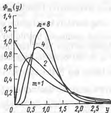
113-rasm. Teng hajmli reaktorlar kaskasida bo'lib turish ehtimolligida F_m(u) zichlikning taqsimlanishi
