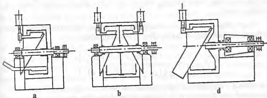
14-rasm. ФГН tipidagi sentrifugalarda rotorning joylashish sxemasi: a — rotor tirgaklar oralig'ida joylashgan; b — tirgaklar oralig'ida ikkita rotor joylashgan; d — rotor qiya tarzda joylashgan.
