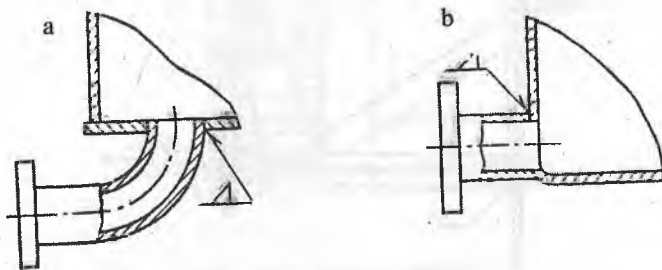
107-rasm. Quyiladigan shtutserlarni payvandlash:
