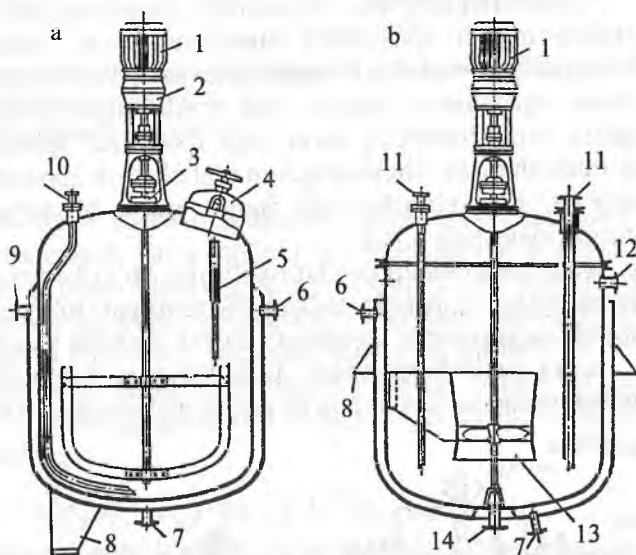
7-rasm. Aralashtirgichli reaktorlar:
