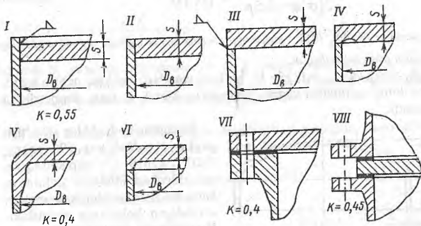
94-rasm. Obechaykalar yassi (tekis) tublarni biriktirish varianti va tub konstruksiyasi koeffitsienti K ning ahamiyati
