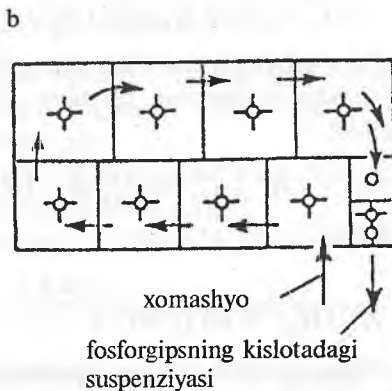
9-rasm. Ekstraksiyon fosfor kislotasi ishlab chiqarish uchun reaktorlar:
