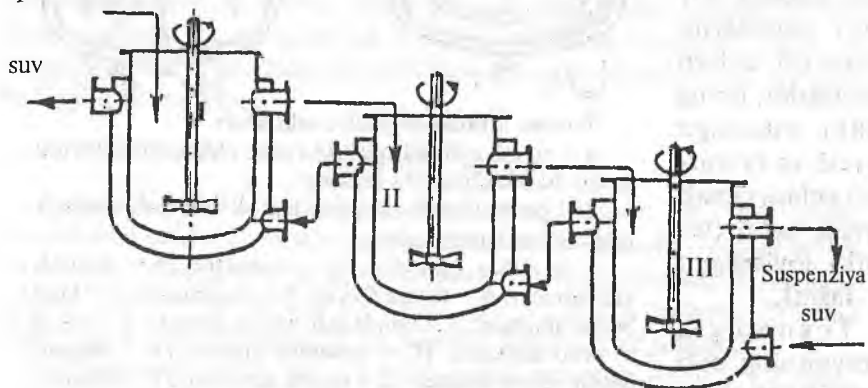
8-rasm. Aralashtirgichlari bor apparatlar termasi (kaskadi).
