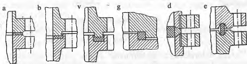
98-rasm. Flanesli biriktiruvchilarni zichlovchi yuzalarining turi:
