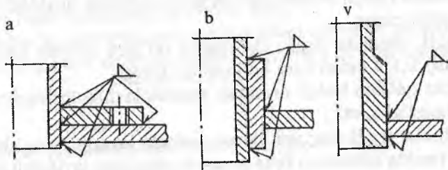
108-rasm. Teshiklarni mustahkamlash usullari: a — yassi halqalar; b — vtulka; v — yo'g'onlashtirilgan shtutser
